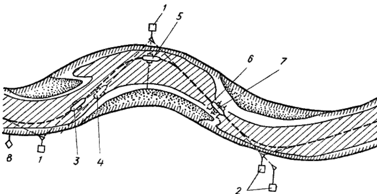
Рис. 26. Схема использования береговых знаков судоходной обстановки: 1 — перевальный знак; 2 — створный знак; 3 — судно на правильном курсе; 4 — судно сошло с правильного курса; 5 — судно на траверзе перевального знака; 6 — каменистый перекат; 7 — судно на линии створа; 8 — ходовой знак
