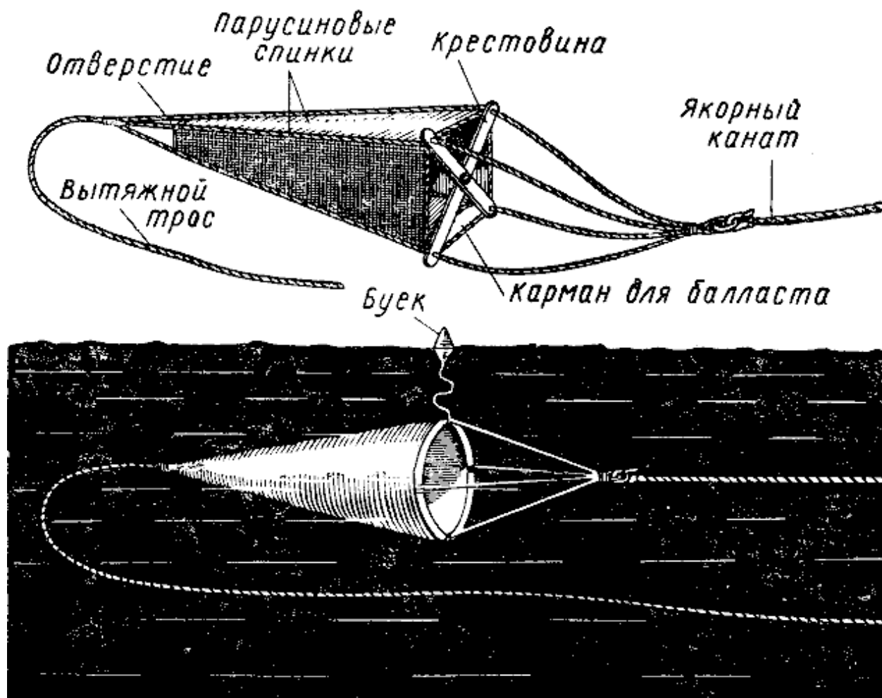
Рис. 129. Плавучие якоря
