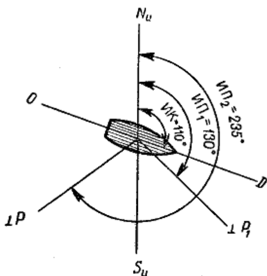
Рис. 41. Графическое определение истинного курса судна и истинного пеленга на предмет
