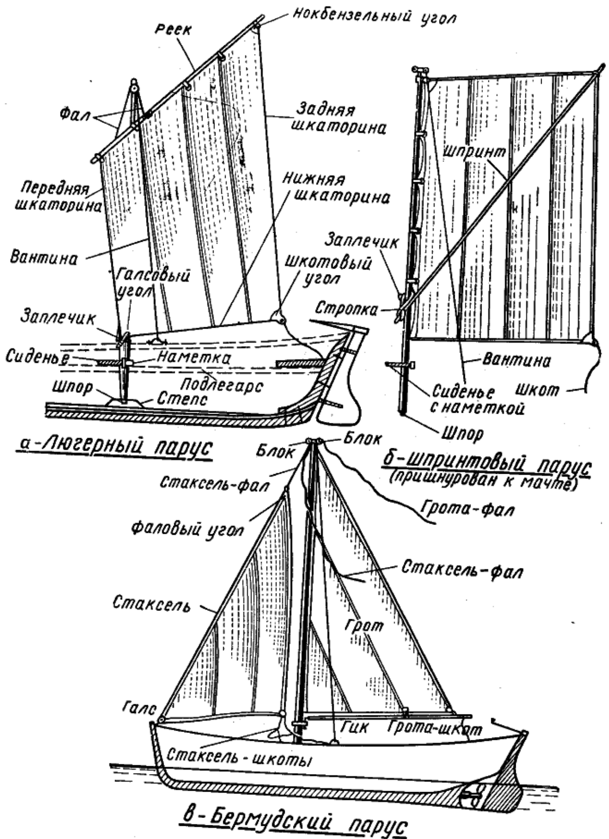
Рис. 144. Детали парусного вооружения
