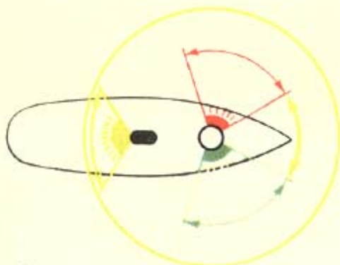
План расположения сигнальных огней на судне, производящем лов рыбы
