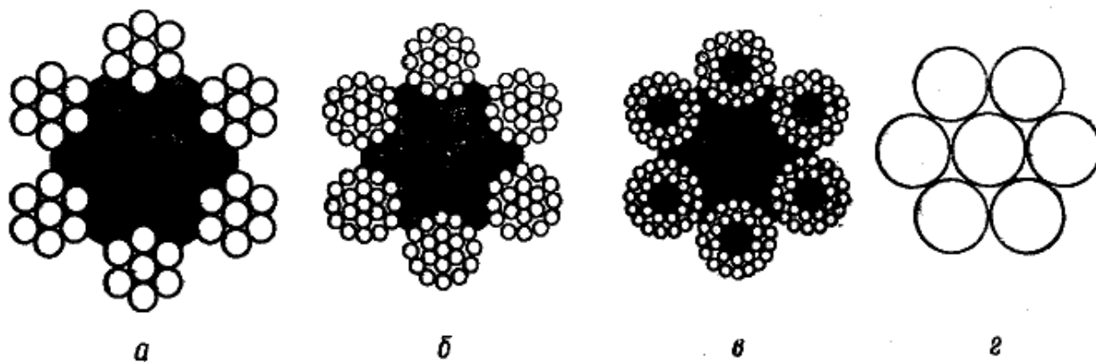
Рис. 151. Стальные тросы: а — жесткий; б — полужесткий; в — гибкий; г — бензель
