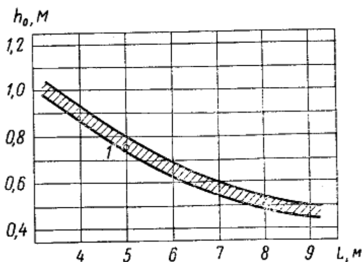
Рис. 90. Зависимость начальной метацентрической высоты от длины судна
