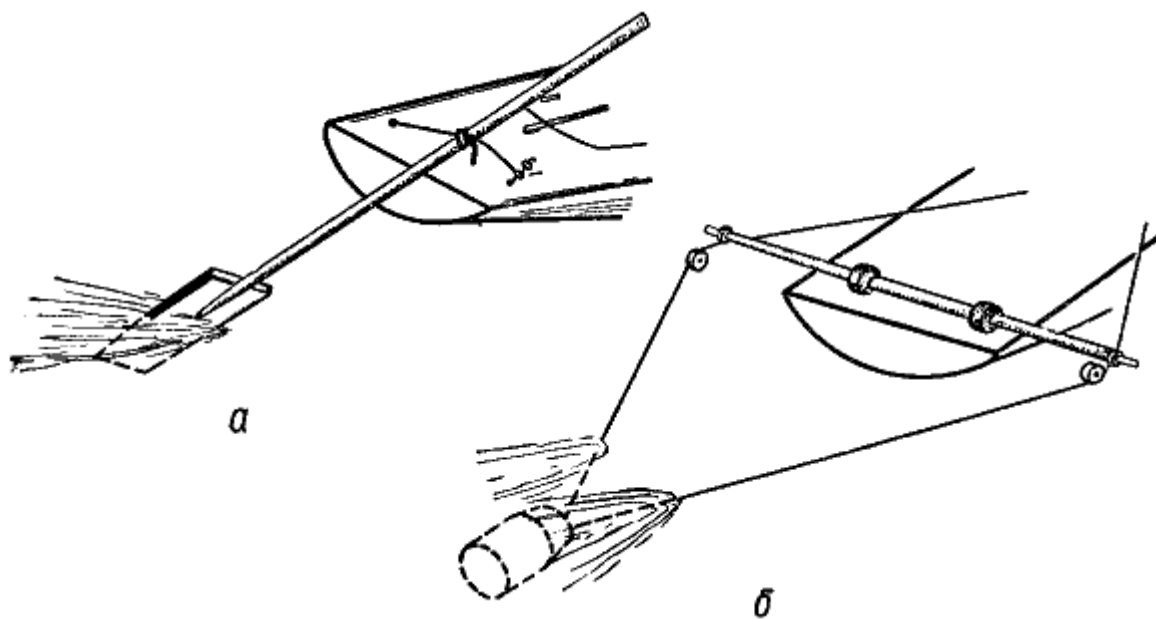
Рис. 134. Управление судном при аварии с рулем: а — кормовым веслом; б—буксировкой предметов
