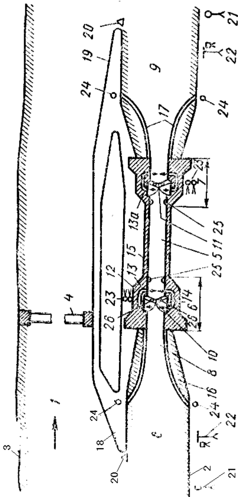
Рис. 30. Общая схема шлюза и подхода к нему: 1 — река; 2 — правый берег; 3 — левый берег; 4 — плотина; 5 — камера шлюза; 6 — верхняя голова шлюза; 7 — нижняя голова шлюза; 8 — верхний подходный канал; 9 — нижний подходный канал; 10 — верхние ворота; 11 — нижние ворота; 12 — шкафная ниша для помещения створок открытых ворот; 13 — короткая водопроводная галерея для наполнения камеры шлюза; 13а — водопроводная галерея для опорожнения камеры шлюза; 14 — затвор водопроводной галереи; 15 — стенки камеры шлюза; 16 — верхние направляющие палы-эстакады; 17 — нижние направляющие палы-эстакады; 18 — верхнее разделительное сооружение; 19 — нижнее разделительное сооружение; 20 — белый бакен; 21 — знак «Сигнал»; 22 — семафор или светофор дальнего действия; 23 двухзначные светофоры, разрешающие или запрещающие выход из камеры; 24 — ограничительные огни на подходах к шлюзу; 25 — столовые огни на стенках камеры шлюза; 26 — огни на створках ворот шлюза
