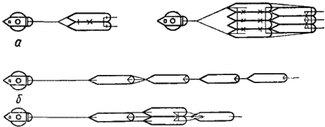
Рис. 109. Формирование составов: а — по течению; б — против течения
