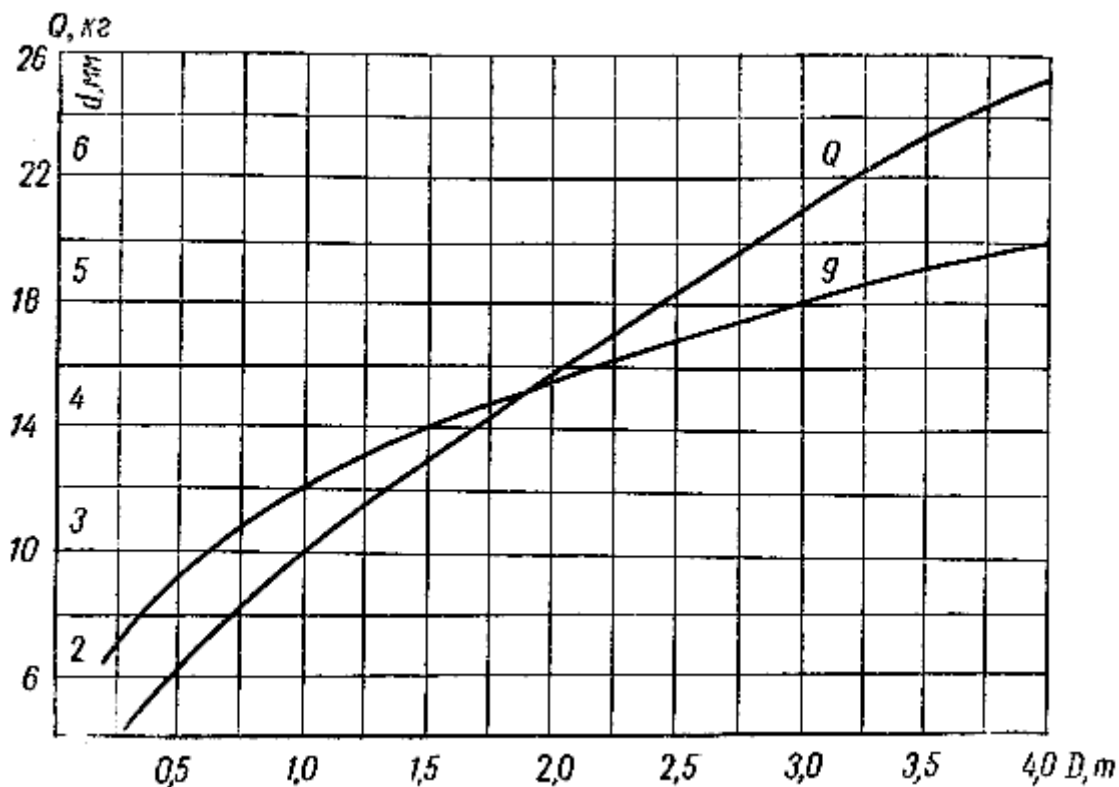
Рис. 114. График для определения веса якоря ( Q ) и калибра якорной цепи ( g )
