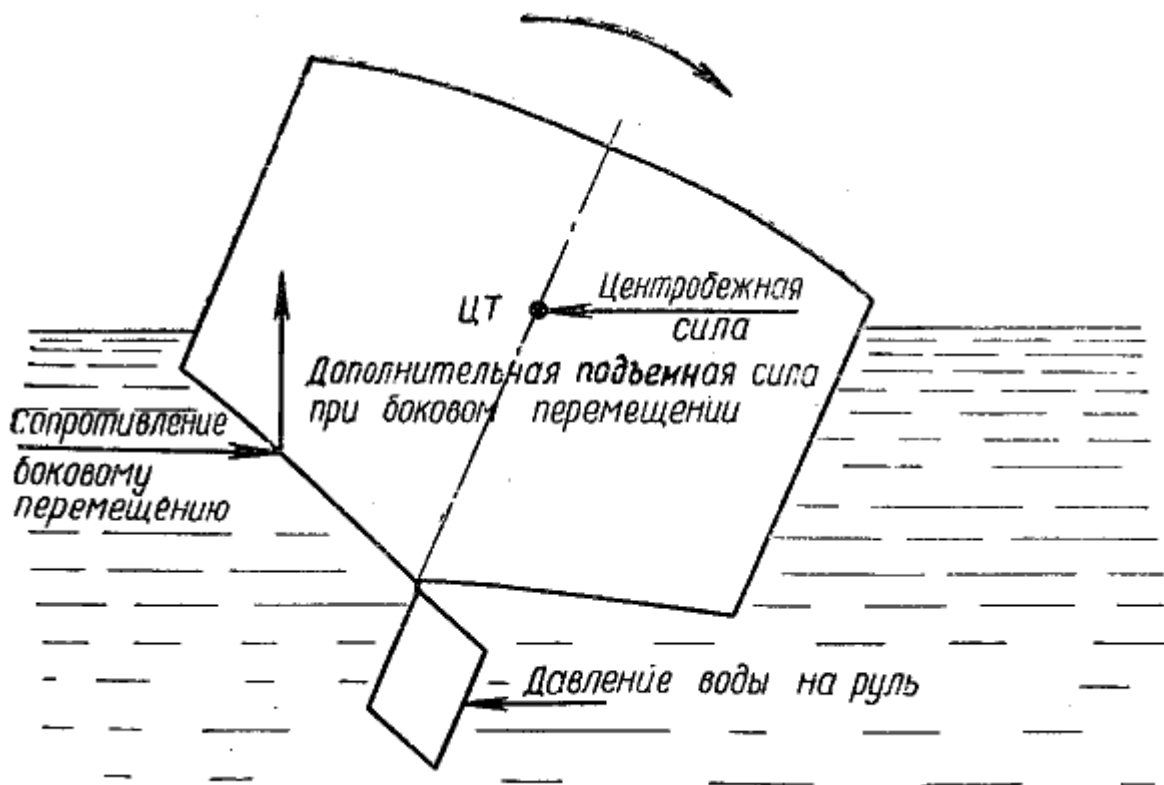
Рис. 97. Действие подъемной силы глиссирующего судна при боковом перемещении
