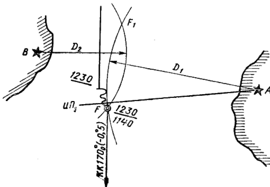
Рис 51 Определение места судна по двум расстояниям до двух предметов
