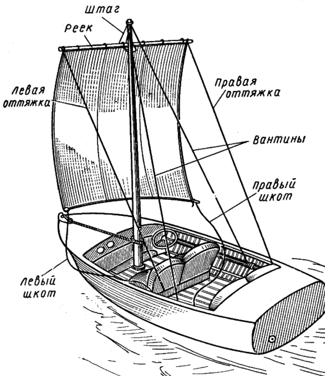
Рис. 145. Аварийный прямой парус
