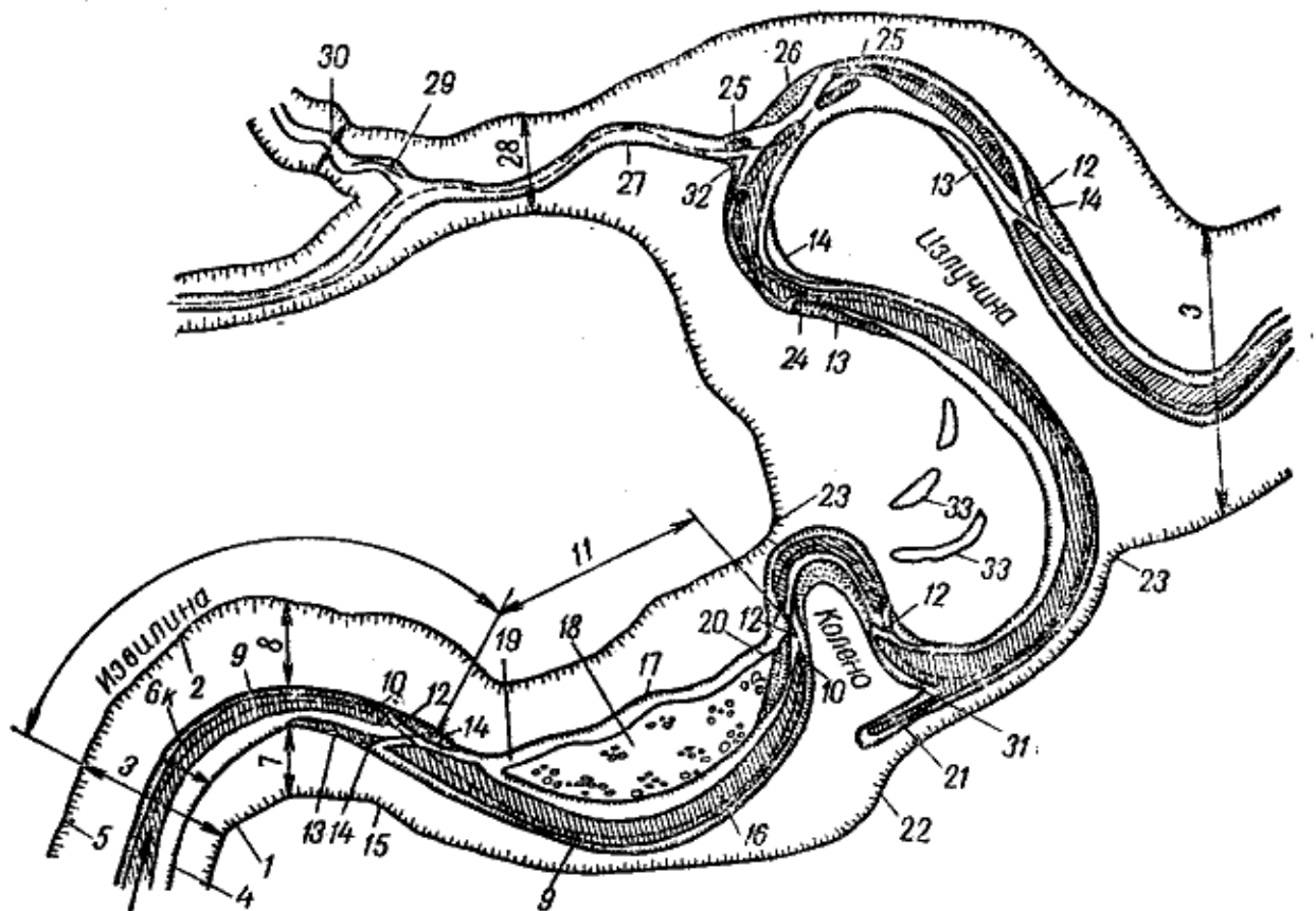
Рис. 8. Схема извилистых участков рек: 1 — правый коренной (незатопляемый) берег; 2 — левый коренной берег; 3 — ширина долины; 4 — правый меженный берег; 5 — левый меженный берег; 6 — ширина меженного русла; 7 — правая пойма; 8 — левая пойма; 9 — яр; 10 — нижнее плечо яра; 11 — верхнее плечо яра; 12 — пережат; 13 — верхняя коса (пески); 14 — нижняя коса (пески); 15 — гребень пережата; 16 — коренное русло; 17 — неходовая воложка; 18 — остров; 19 — приверх острова; 20 — ухвостье острова; 21 — затон; 22 — защитная линия ледорезов; 23 — рынок; 24 — перевал; 25 — осередок; 26 —
