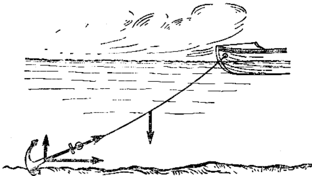
Рис. 115. Стоянка на якорю
