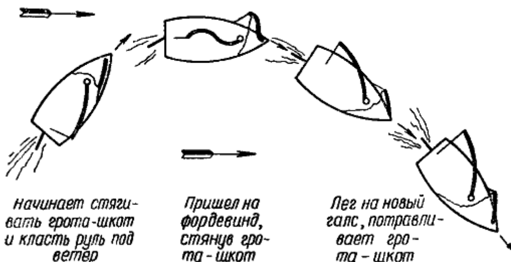
Рис. 141. Поворот через фордевинд
