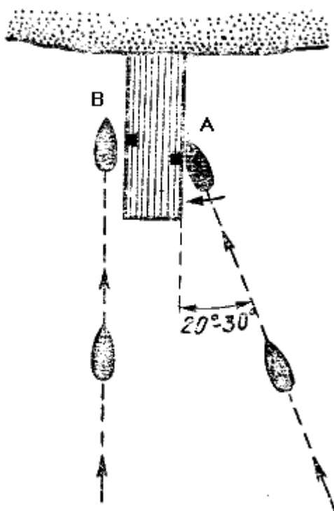
Рис. 118 Подход катера с винтом правого вращения к причалу
