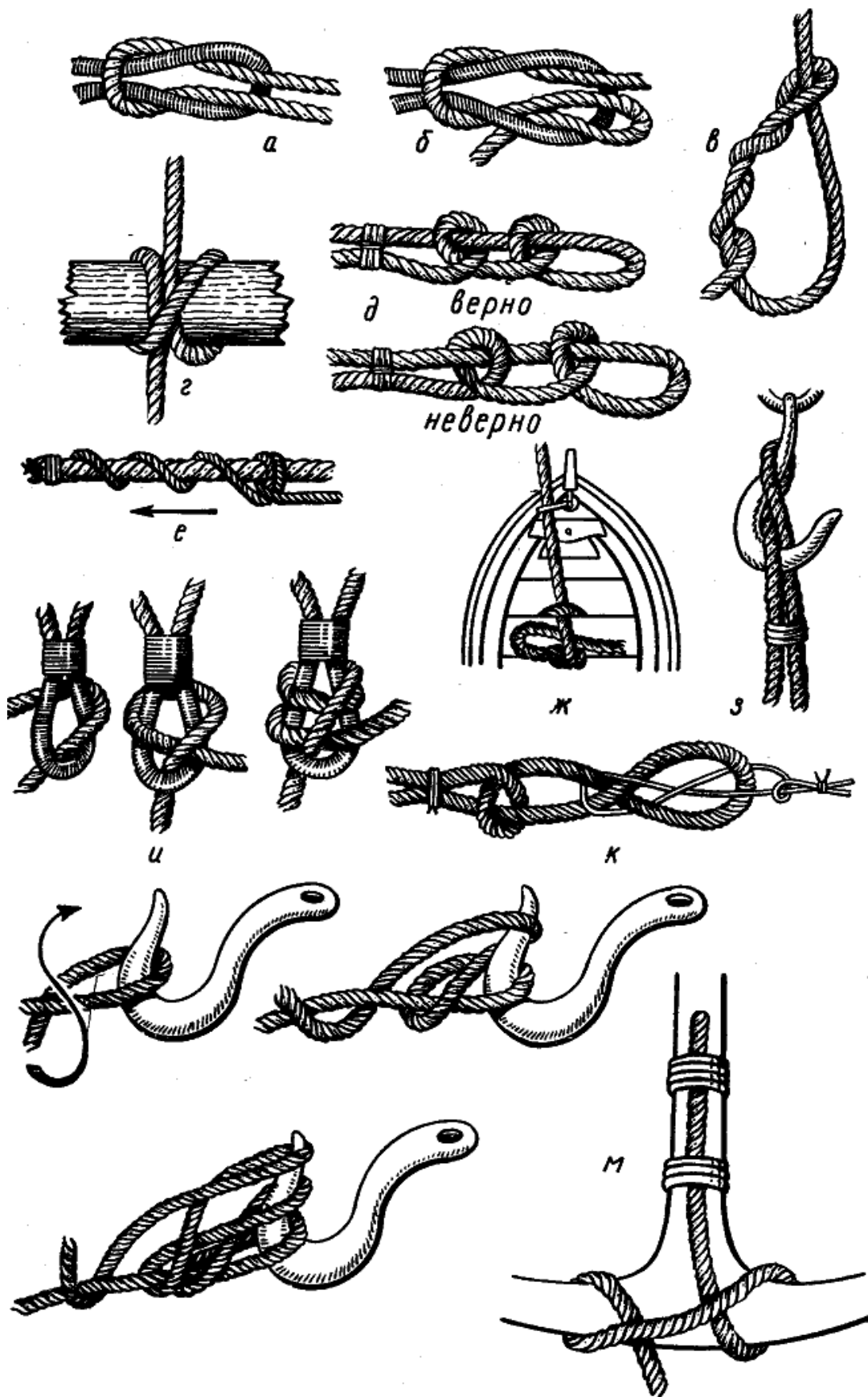
Рис. 153 Морские узлы: а — прямой, б — рифовый, в — удавка, г — выбленочный; д — простой штык; е — стопорный узел; ж — шлюпочный узел; з — гачный узел; и — шкотовый (слева) и брамшкотовый (справа); к — плоский узел; л — буксирный, м — буйрепный узел
