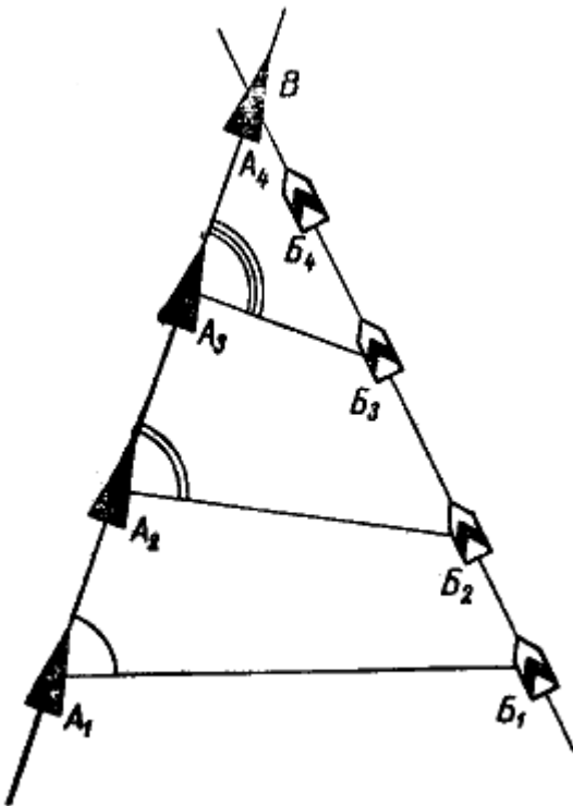
Рис. 174. Случай уменьшения пеленга
