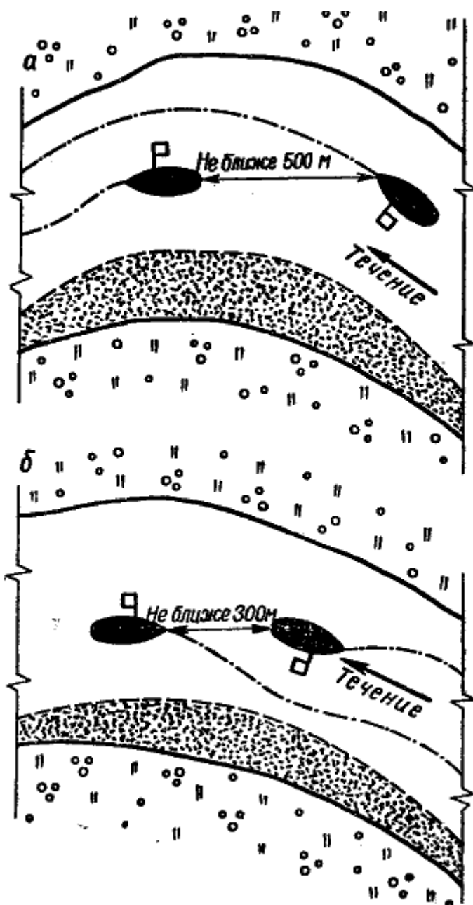
Рис. 170. Обмен сигналами при обгоне судов
