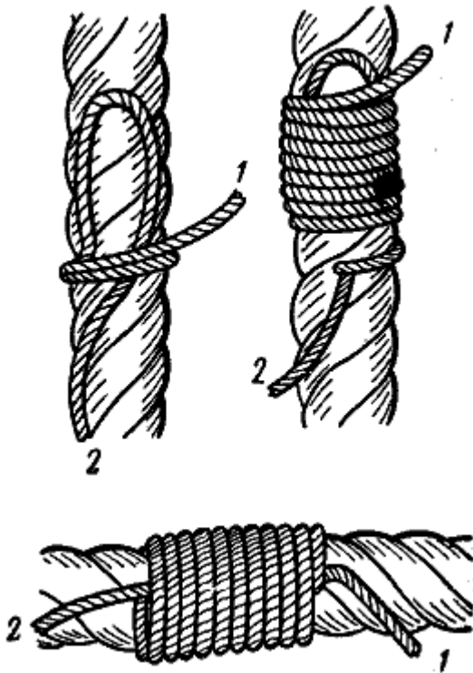
Рис. 156. Простая марка: 1 — ходовой конец; 2 — коренной конец
