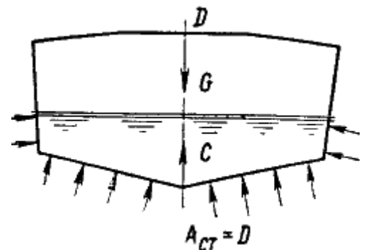
Рис. 86. Статические силы, действующие на судно в состоянии покоя
