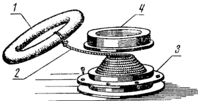
Рис. 163. Спасательное устройство: 1 — плавучее кольцо; 2 — плавучий лить; 3 — бухта, уложенная в специальный корпус; 4 — крышка для закрытия спасательного устройства
