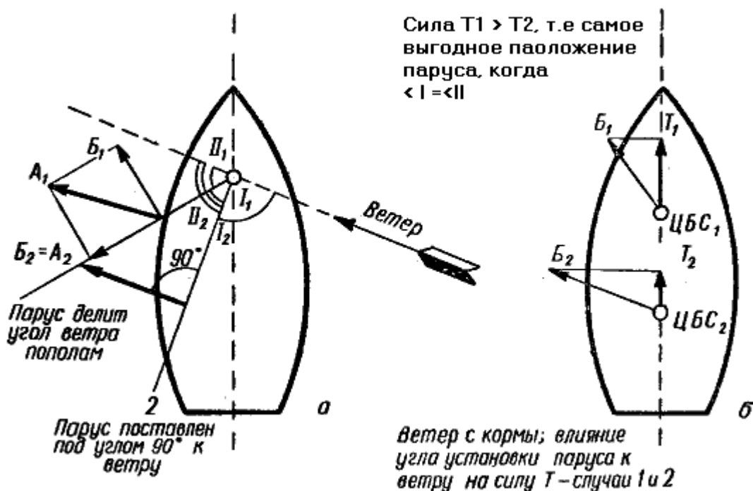
Рис. 138. Силы, действующие на парус и судно при ветре с кормовых углов
