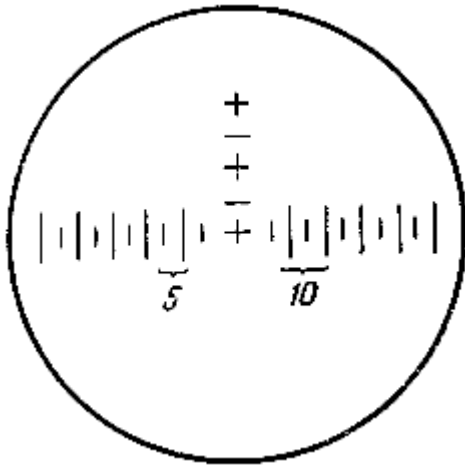
Рис. 74. Сетка призматического бинокля
