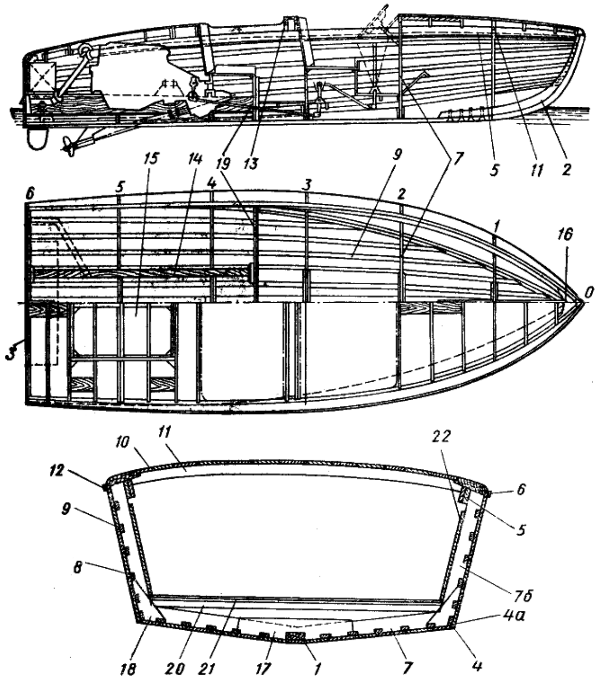
Рис. 3. Конструктивный чертеж быстроходного катера: 1 — киль; 2—форштевень; 3—транец; 4 — скуловой стрингер; 4а — скуловая планка; 5—привальный брус; 6—планширь (ватервейс); 7 — флортимберс; 7б — топтимберс; 8—наружная обшивка; 9 — пазовая рейка; 10 — настил палубы; 11 — бимс; 12 — буртик; 13 — комингс; 14 — брус фундамента; 15 — надмоторный люк; 16 — брештук; 17 — кница; 18 — скуловая кница; 19—водонепроницаемая переборка; 20 — лежни слани; 21 — слань; 22— внутренняя обшивка
