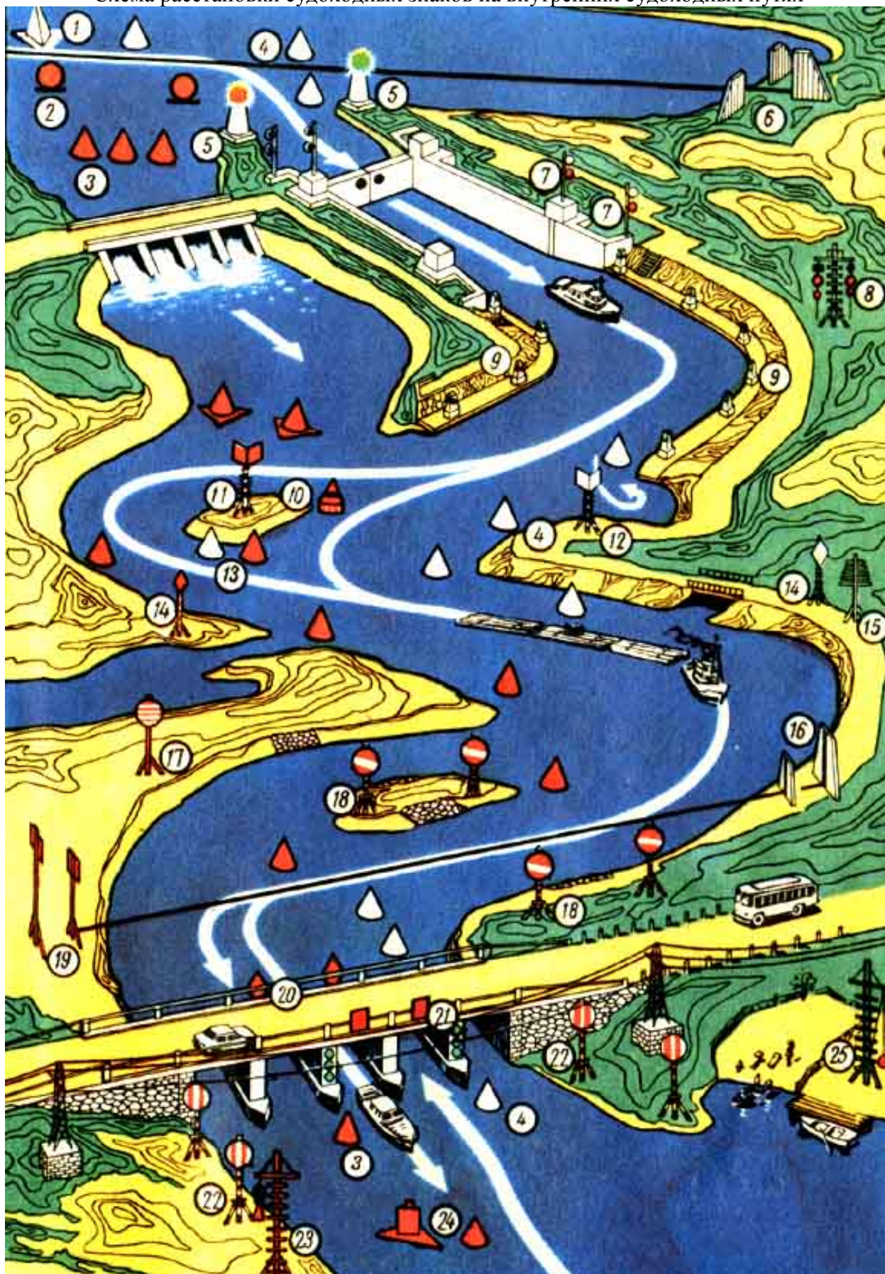
Схема расстановки судоходных знаков на внутренних судоходных путях
