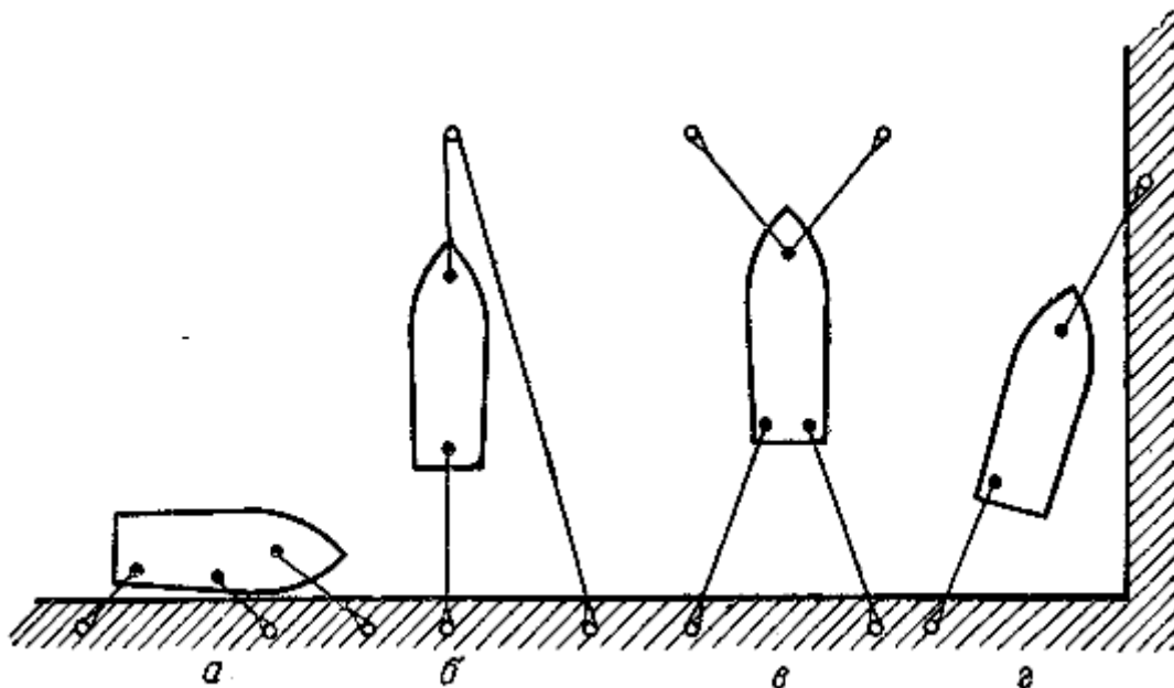
Рис. 121. Стоянка судов
