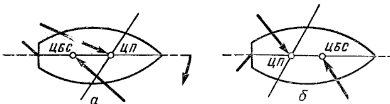
Рис. 104. Увальчивость и рыскливость судна: а — увальчивость; б — рыскливость
