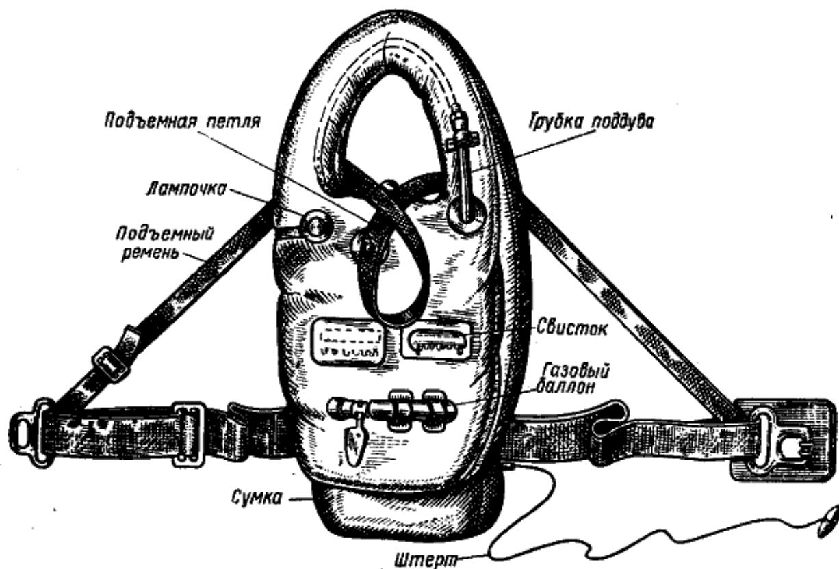
Рис. 161. Надувной спасательный нагрудник
