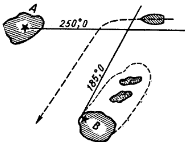
Рис. 53. Опасные пеленги
