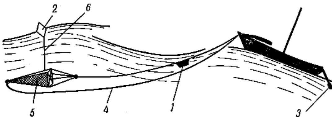
Рис 128 Шлюпка на плавучем якорю: 1 — мешок с маслом; 2 — буюк; 3 — рулевое весло; 4 — трос для выбирания якоря; 5 — якорь; 6 — буйреп
