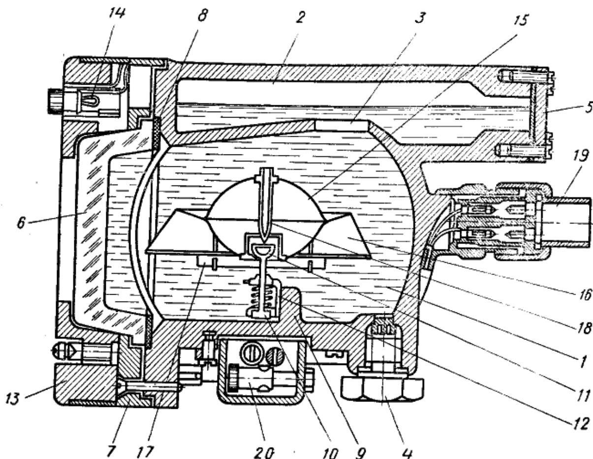
Рис 68 Котелок компаса КИ-11: 1 — основная камера, 2 — дополнительная камера, 3 — перепускное отверстие, 4 — отверстие для доливки и заливки жидкостей, 5 — крышка дополнительной камеры, 6 — выпуклое стекло переднего отверстия котелка, 7 — прижимное стекло, 8 — пробковая прокладка, 9 — кронштейн, 10 — колонка, 11 — топка, 12 — амортизационная пружина, 13 — наружное кольцо, 14 — электрическая лампочка, 15 — поплавок; 16 — конический обод со шкалой, 17 — магнитные стрелки, 18 — стальная шпилька, 19 — вилка электроосвещения, 20 — девиационный прибор
