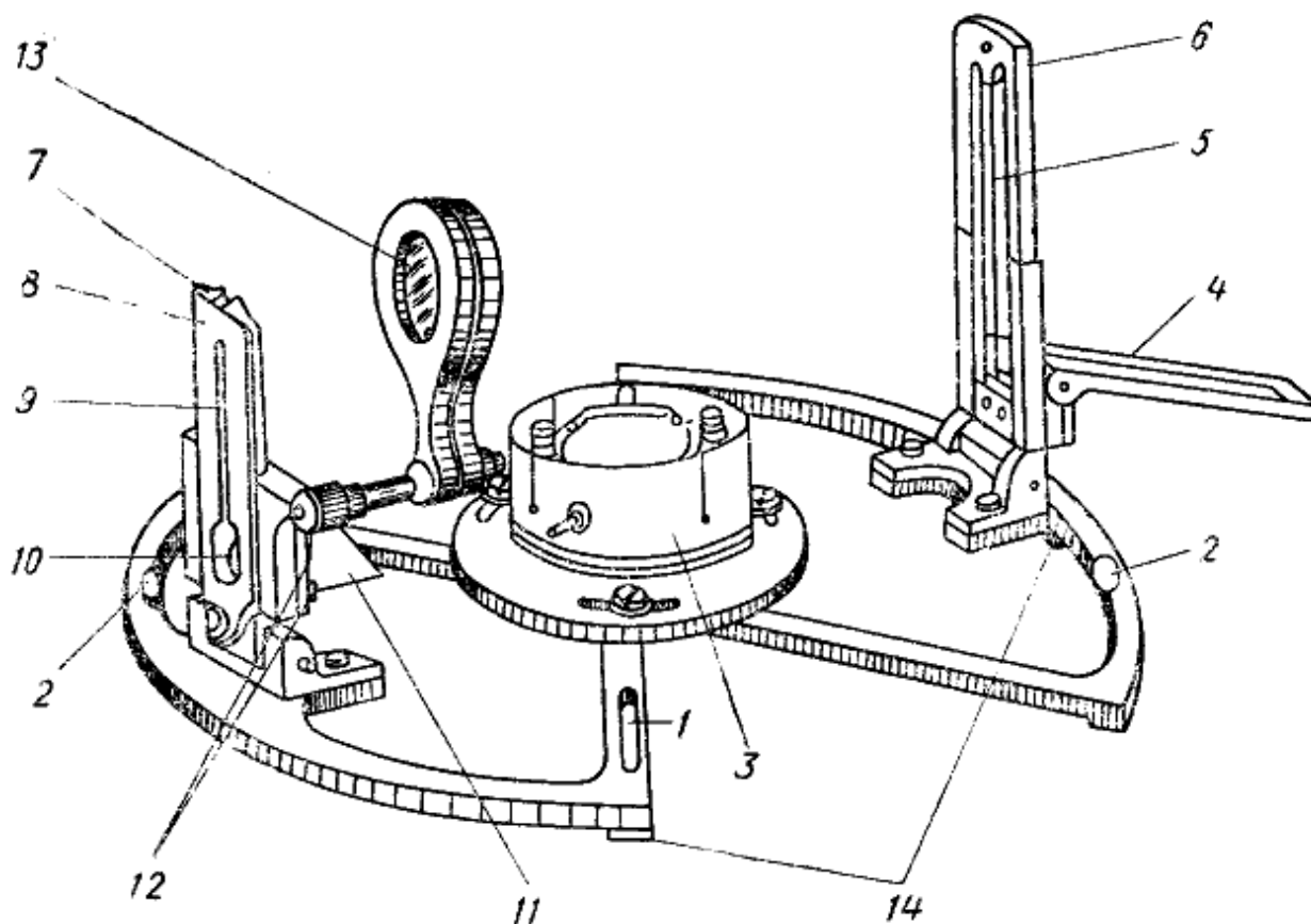
Рис 64. Пеленгатор 127-миллиметрового компаса: 1 — стойка для проворачивания пеленгатора; 2—индекс; 3 — чашка пеленгатора; 4 — откидное зеркало; 5 — пеленгаторная нитка; 6 — предметная мишень; 7 — глазная мишень; 8 — откидной щиток; 9 — щель для дневного пеленгования; 10 — призма, 11 — откидной щиток призмы; 12—винтики, крепящие оправу призмы; 13 — цветные стекла; 14 — лапки
