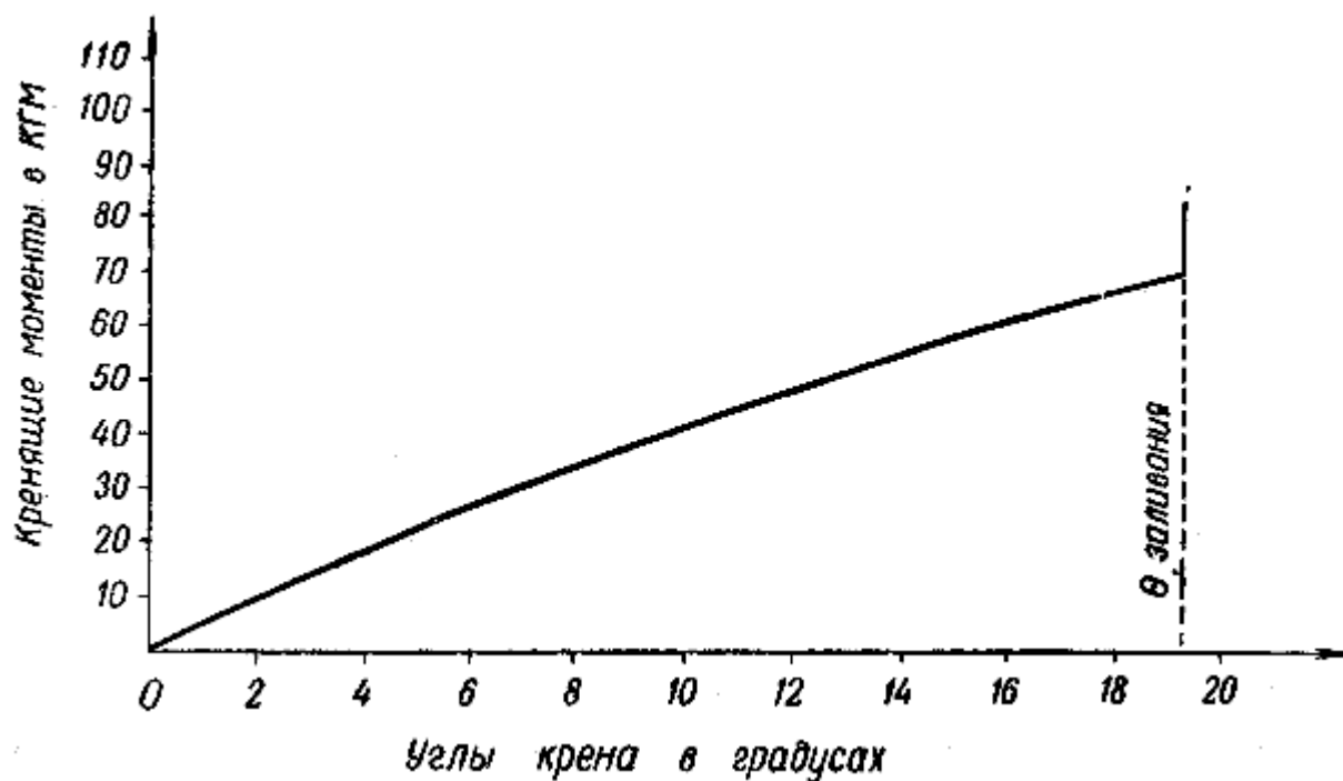
Рис 91. Диаграмма статической остойчивости
