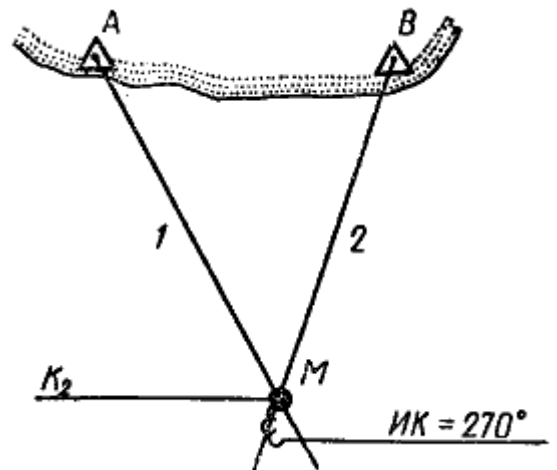
Рис. 49. Определение места судна по пеленгам двух предметов
