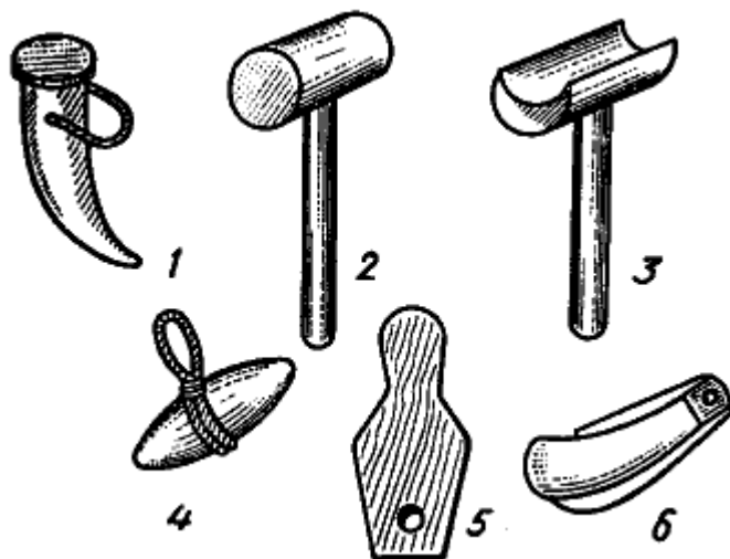
Рис. 152. Такелажный инструмент 1 — свайка, 2 — мушкель, 3 — полумушкель, 4 — драек, 5 — лопатка, 6 — нож
