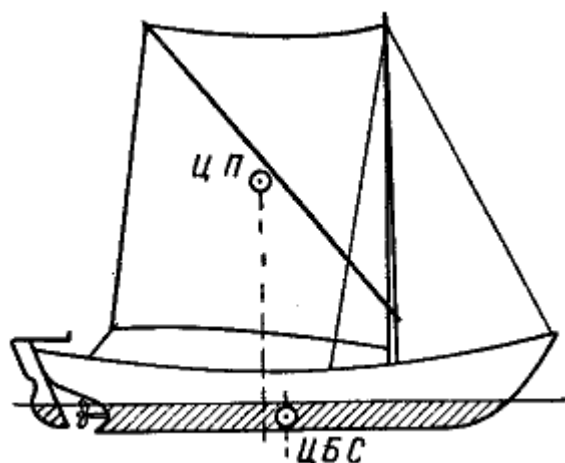
Рис. 139. Положение центра парусности относительно центра бокового сопротивления
