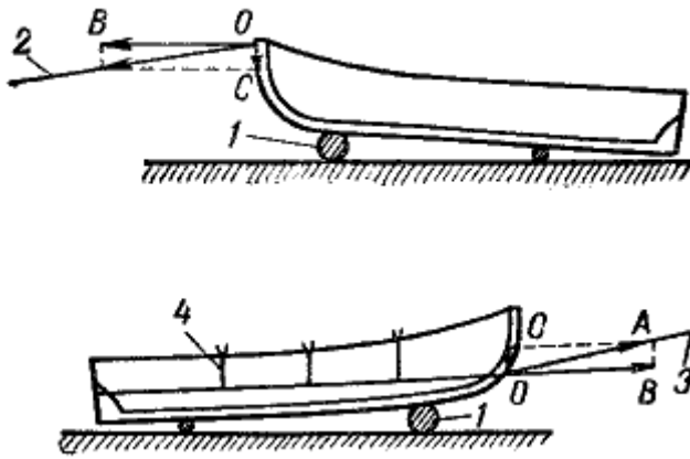
Рис 132. Снятие шлюпки с мели: 1 — круглые бревна; 2 — фалинь; 3 — якорный канат; 4 — штерты, на которых подвешен якорный канат
