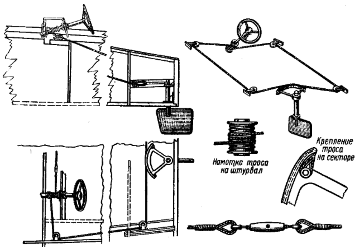
Рис. 99. Рулевое устройство катера
