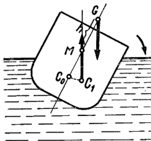
Рис. 94. Случай нестойчивого судна при неустойчивом равновесии
