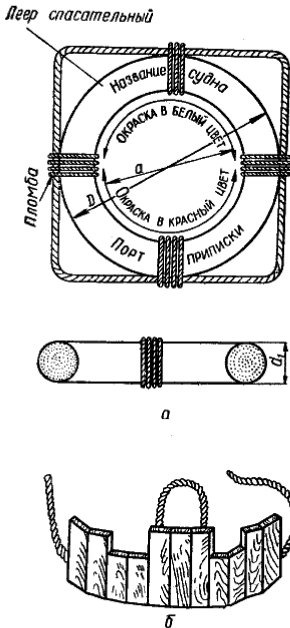
Рис. 159. Спасательные средства: а — спасательный круг; б — спасательный пояс
