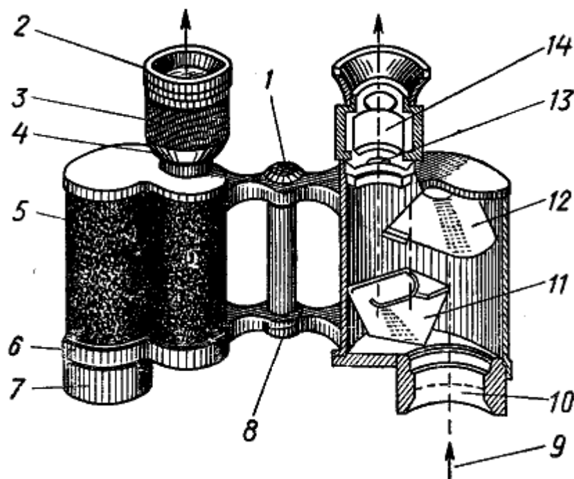
Рис. 73. Призматический бинокль: 1 — винт шайбы шарнира; 2 — наглазник; 3 — кольцо с накаткой; 4 — диоптрийное стекло; 5 — окулярная крышка; 6 — крышка объектива; 7 — наружное кольцо оправы объектива; 8 — шарнир; 9 — ход лучей; 10 — объектив; 11 — призма объективная; 12 — призма окулярная; 13 — линза; 14 — окуляр
