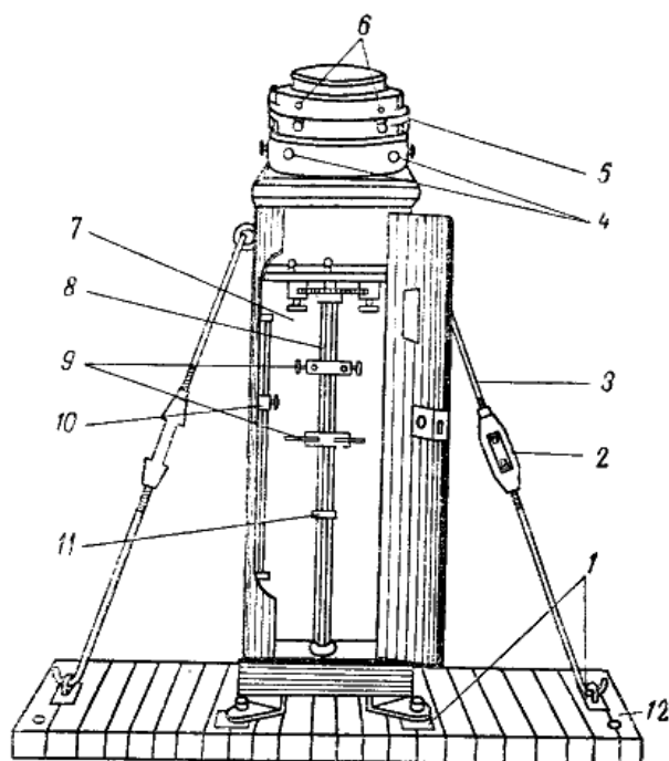
Рис. 65. Нактоуз: 1 — палубные планки; 2 — талреп; 3 — бакштаг; 4 — бруски мягкого железа; 5 — шейка; 6 — клеммы пружинного подвеса; 7 — девиационный прибор; 8 — труба; 9 — гнезда для магнитов; 10 — ползун с барашком; 11 — кольцо, закрепляющее креповой магнит; 12 — подушка
