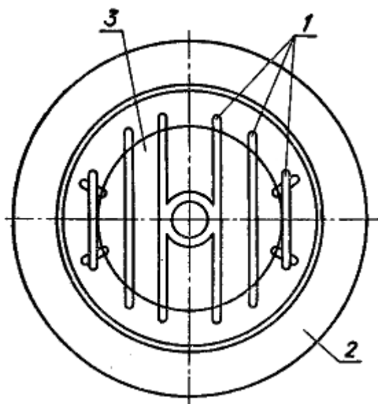
Рис. 62 Картушка магнитного компаса: 1 — магнитные стрелки; 2 — картушка; 3 — поплавок
