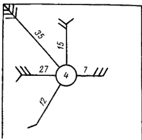
Рис. 78 Диаграмма розы ветров
