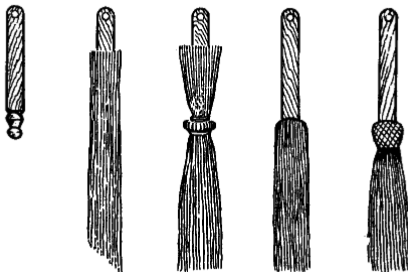
Рис. 158. Изготовление швабры (последовательные приемы изготовления)
