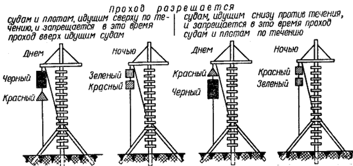
Рис. 23. Семафорные мачты
