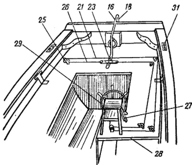
Рис. 5. Рулевое устройство моторного барказа БМ-16: 16 — рычажный румпель; 18 — баллер; 21 — штуртрос; 23 — планка, движущаяся в прорези румпеля; 25 — одношківные ролики; 26 — талреп; 27 — штурвальная рама; 28 — банка; 31 — киповая планка
