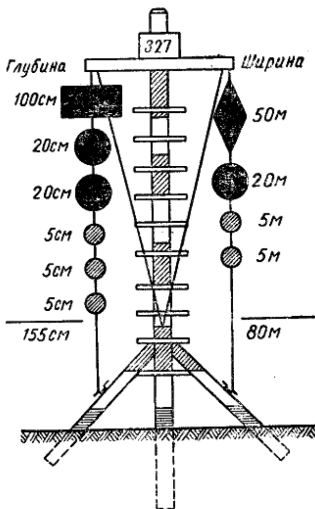
Рис. 21. Сигнальная мачта левого берега
