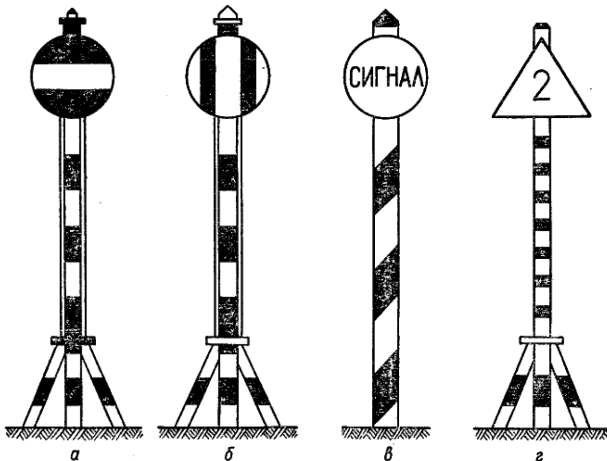
Рис. 22. Путьевые береговые знаки: а — подводного перехода (кабели, трубопроводы и т. д.); б — знак надводных переходов проводов; в — знак сигнала; г — рейдовый знак
