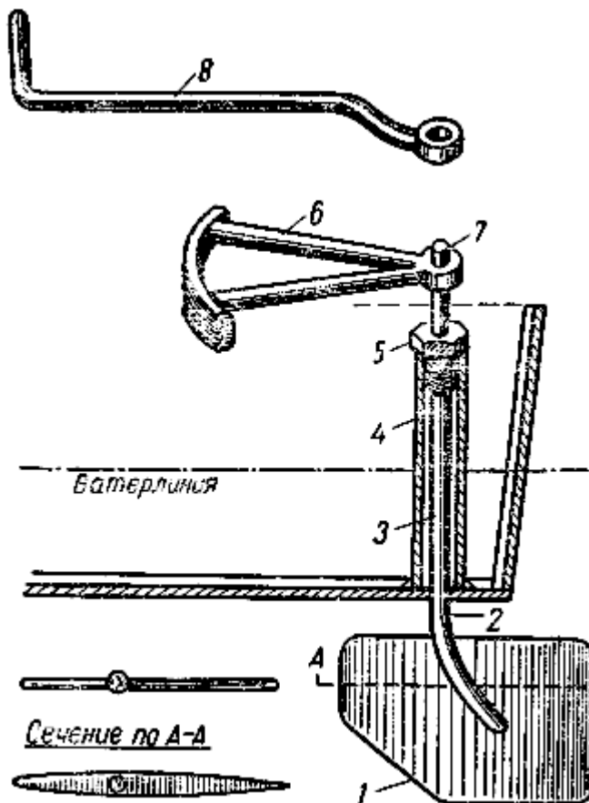
Рис. 102. Конструкция руля 1 — перо руля; 2 — баллер; 3 — труба гельмпорта; 4 — втулка трубы гельмпорта; 5 — сальники; 6 — секторный румпель; 7 — квадрат; 8 — продольный румпель
