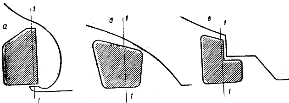
Рис 101. Типы рулей а — обыкновенный; б — балансирующий, в — полубалансирующий
