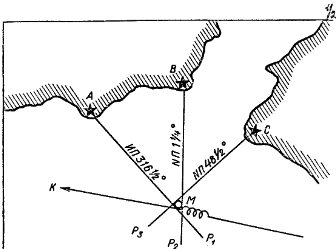
Рис. 50. Определение места судна по пеленгам трех предметов
