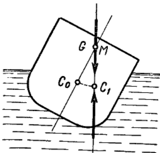
Рис. 93. Случай нестойчивого судна при безразличном равновесии
