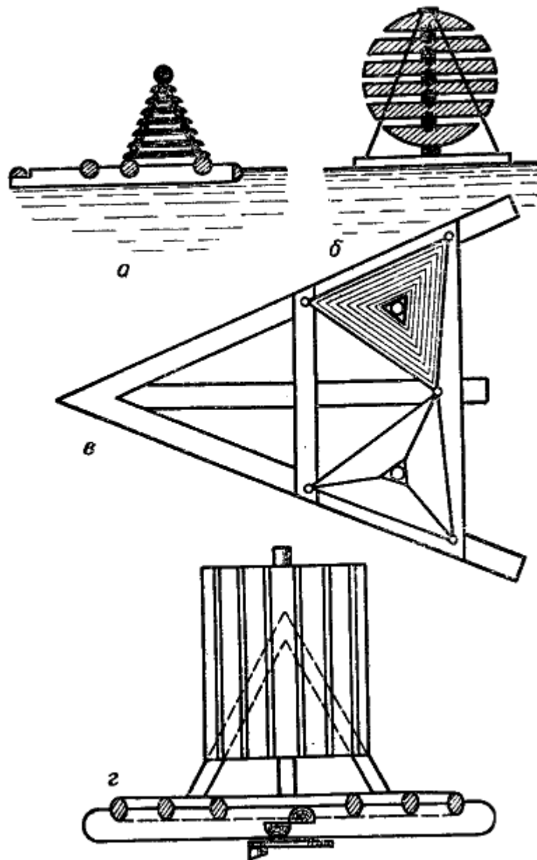
Рис. 19. Бакены: а — красный; б — шаровый, в — спаренный; г — свальный
