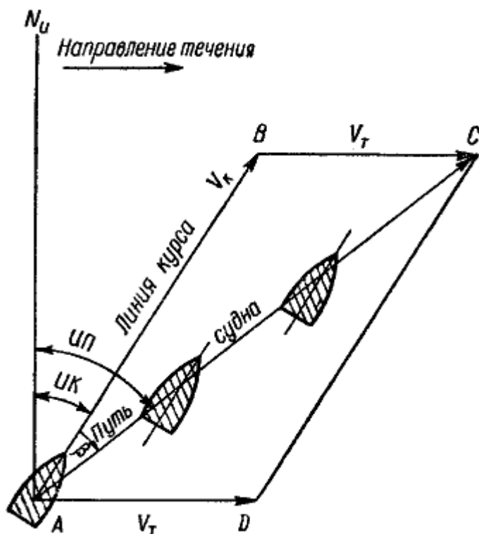
Рис. 45. Плавание судна с учетом течения
