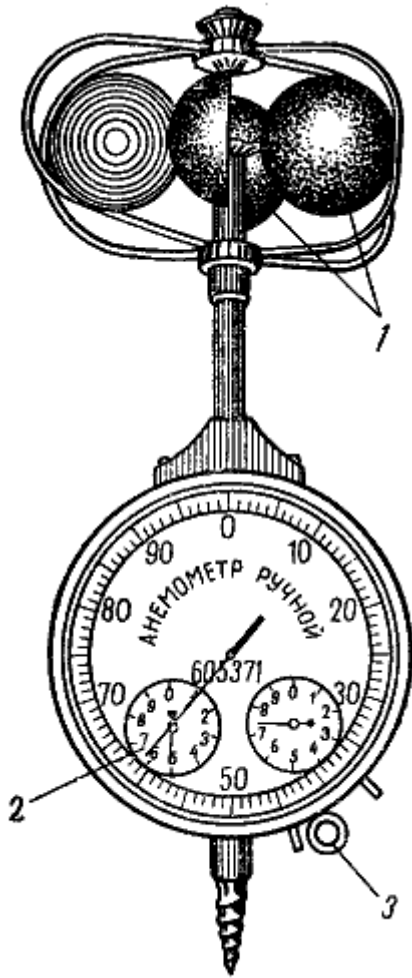
Рис. 84. Анемометр ручной: 1 — полушария крестовины; 2 — отсчет 6560 мм; 3 — арретир
