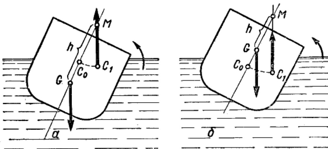
Рис. 92. Случай устойчивого судна
