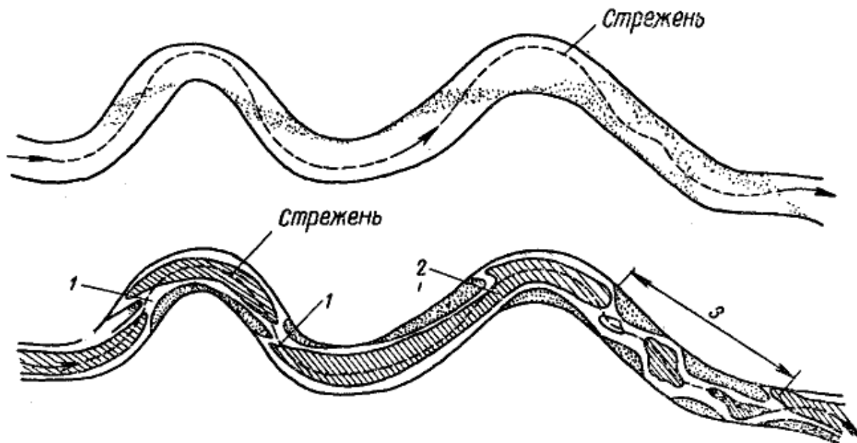
Рис. 14. Перемещение наносов в речном русле и образование перекатов (1, 2, 3) и плесов
