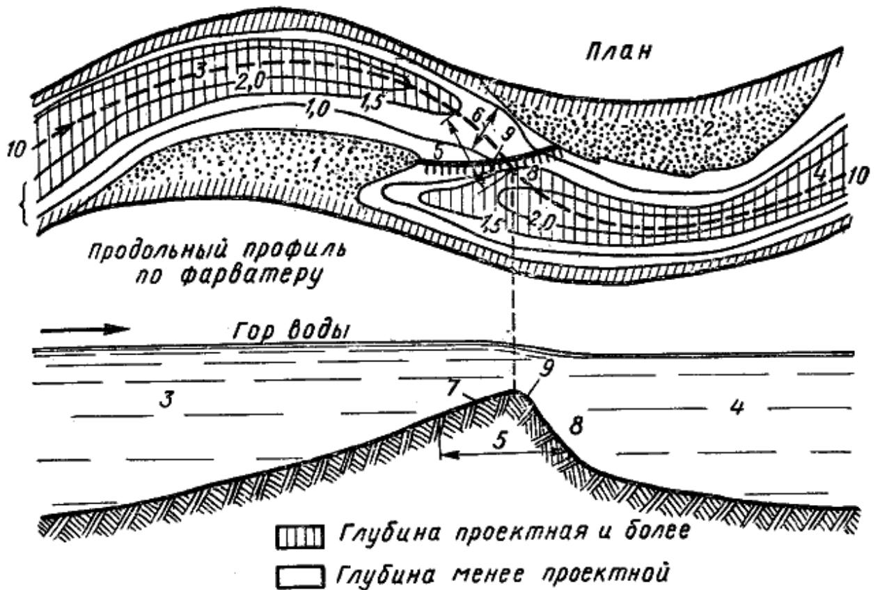
Рис. 17. Перекат: 1 — верхняя коса; 2 — нижняя коса; 3 — верхняя плесовая лощина; 4 — нижняя плесовая лощина; 5 — седловина переката; 6 — корыто переката; 7 — напорный скат; 8 — подвалье переката; 9 — гребень переката; 10 — фарватер
