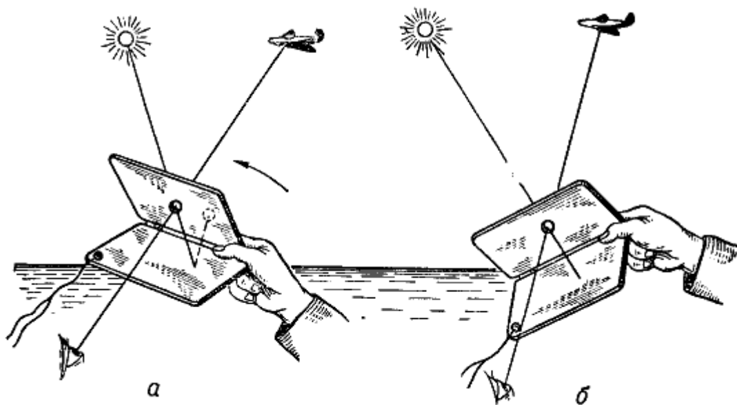
Рис. 149. Использование светосигнального зеркала. а — совмещение солнечного пятна; б — подача сигналов
