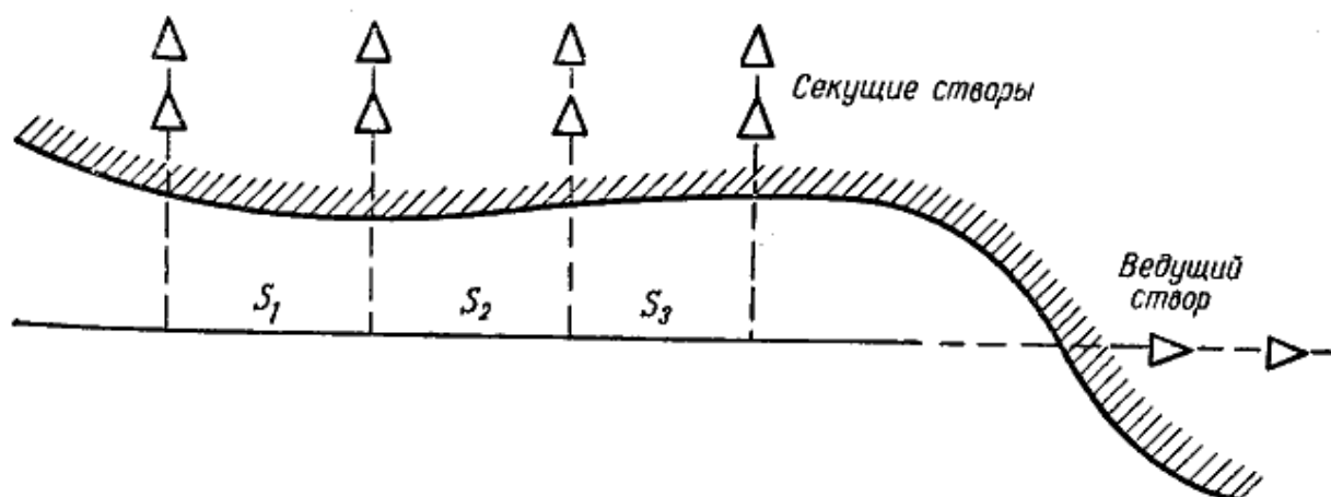
Рис. 59. Схема оборудования мерной линии
