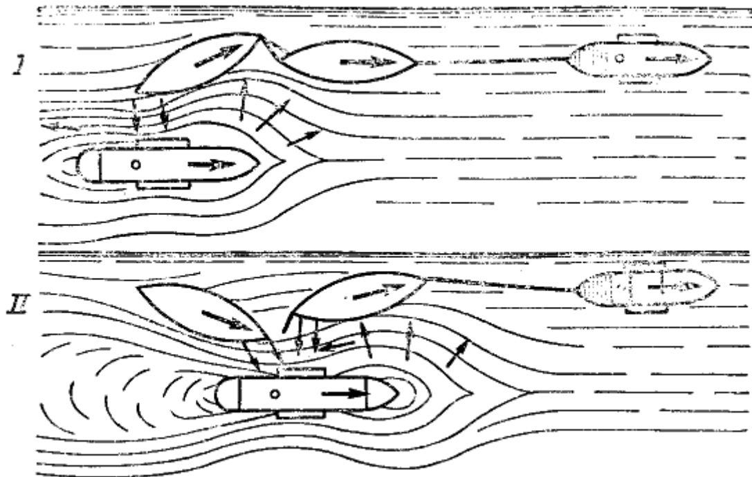
Рис 107. Действие идущего обгоняющего одиночного судна на буксирные суда: I — судно подходит к обгоняемым несамоходным судам; II — судно проходит мимо обгоняемых несамоходных судов
