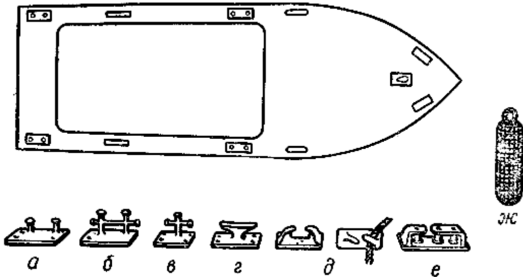
Рис. 117. Швартовные устройства а — обыкновенный кнехт; б, в — крестовые кнехты; г, д, е — киповые планки, ж — кранец мягкий
