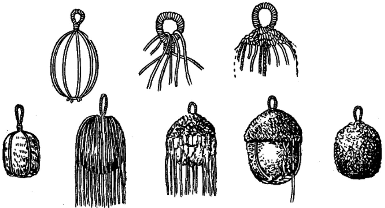
Рис. 157. Изготовление мягкого кранца
