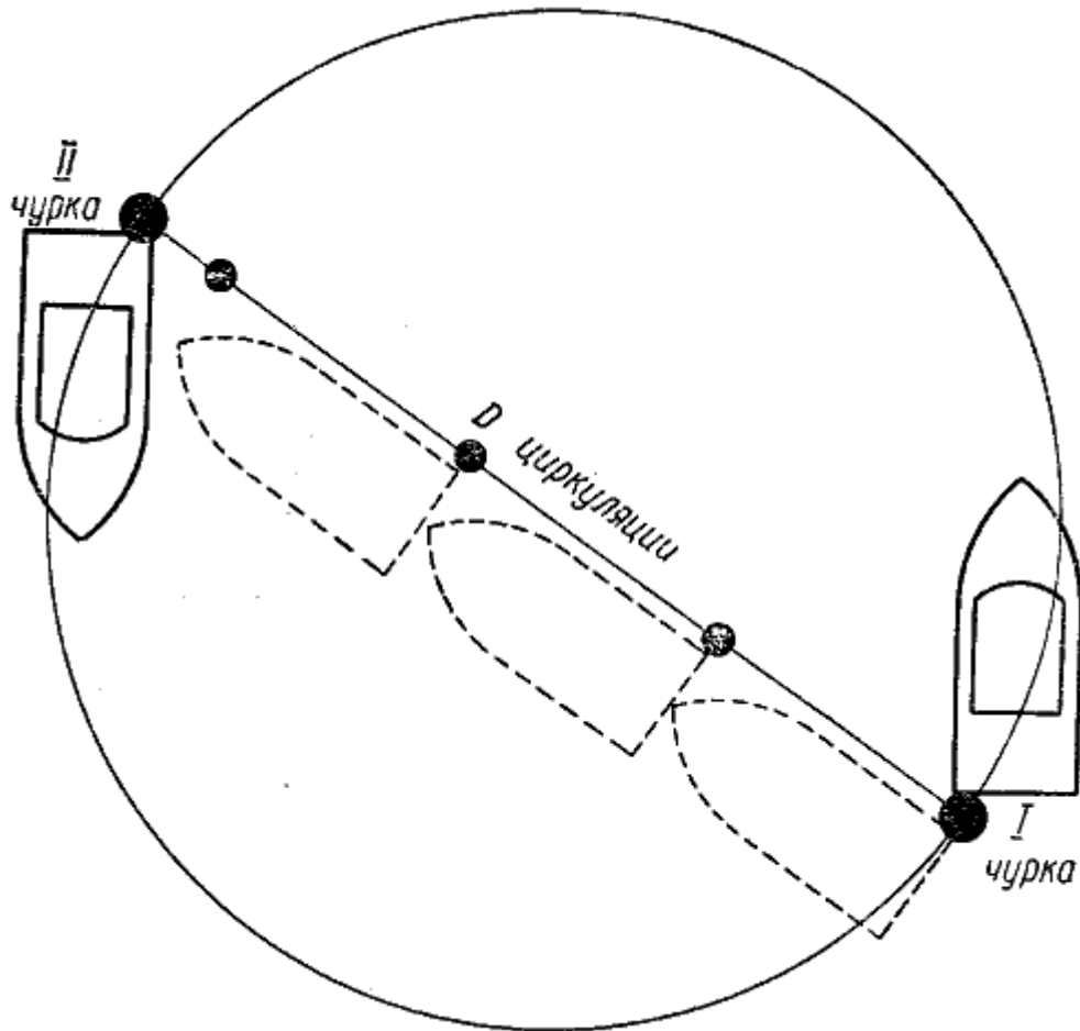
Рис 96. Определение диаметра циркуляции судна
