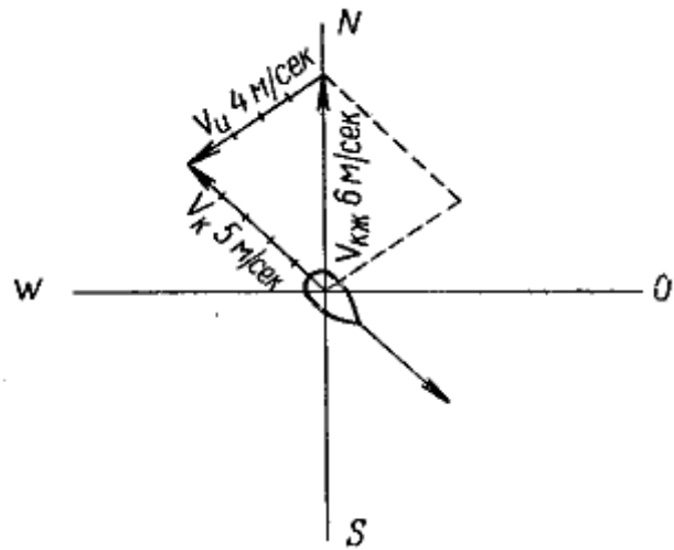
Рис. 85. Графический способ определения истинного ветра на движущемся судне
