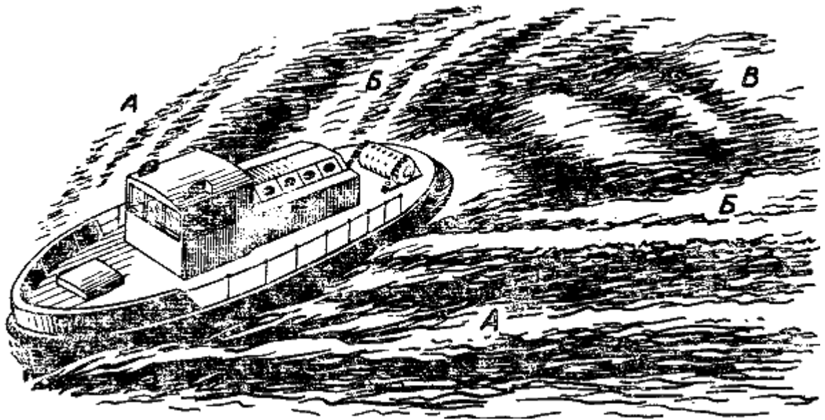
Рис. 105. Схема образования волн при движении судна на спокойной воде А — носовые расходящиеся волны; Б — кормовые расходящиеся волны; В — кормовые поперечные волны
