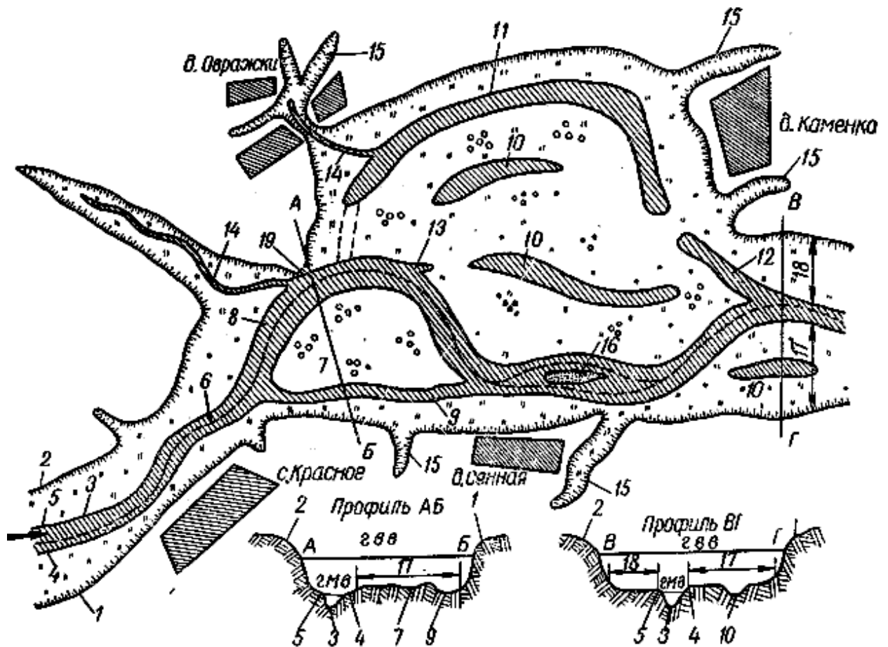
Рис. 7. Схематический план речной долины и русла: 1 — правый коренной (незатопляемый) берег (кряж); 2 — левый коренной берег (кряж); 3 — русло; 4 — правый меженный (затопляемый) берег; 5 — левый меженный берег; 6 — фарватер; 7 — остров; 8 — коренное (ходовое) русло; 9 — воложка (неходовая); 10 — пойменное озеро; 11 — староречье (старица); 12 — затон; 13 — начало прорыва; 14 — приток (речка); 15 — овраги; 16 — осередок; 17 — правая пойма; 18 — левая пойма; 19 — горный рынок (рынок гор); г. в. в. — горизонт высоких вод; г. м. в. — горизонт меженных вод
