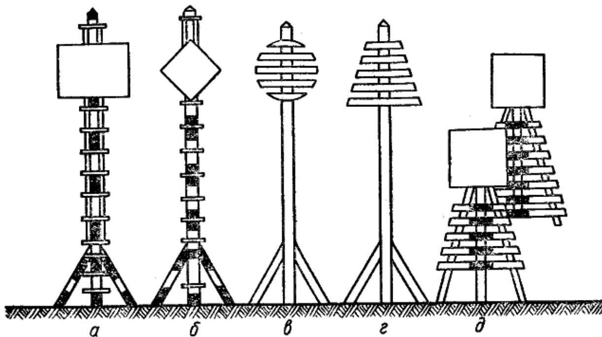
Рис. 20. Знаки, указывающие направление фарватера: а — перевальный знак, б — ходовой знак; в — весенний знак правого берега; г — весенний знак левого берега; д — створы
