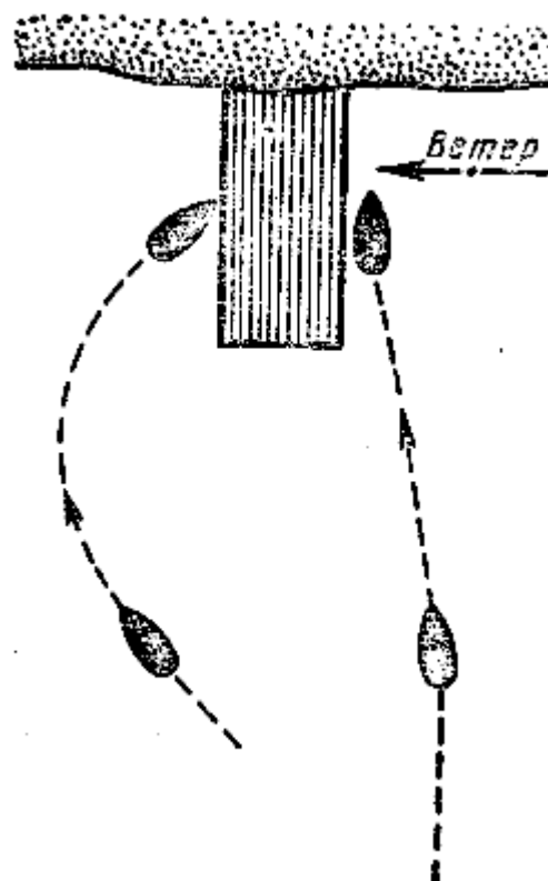
Рис. 119. Подход катера к причалу при наличии ветра
