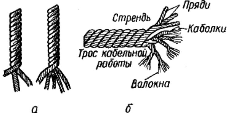
Рис. 150. Тросы: а — трехпрядный и четырехпрядный тросы тросовой работы; б — пеньковый трос кабельной работы и его части
