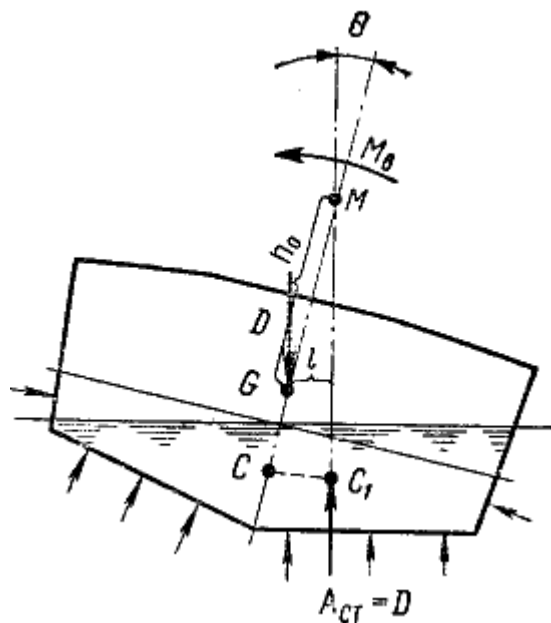
Рис 89 Статические силы, действующие на судно при малых наклонениях
