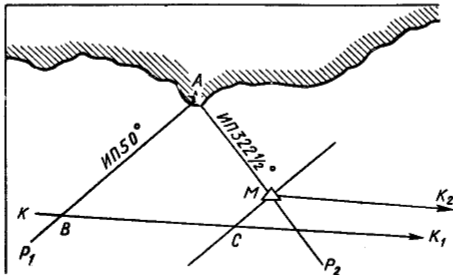
Рис. 48. Определение места судна способом крьюйс-пеленга
