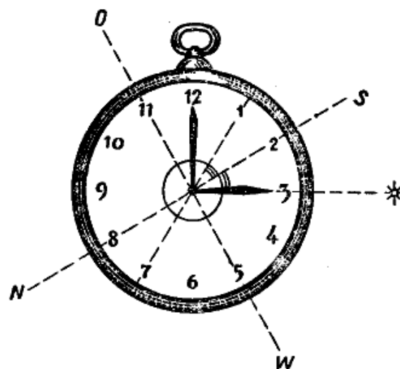
Рис. 58. Определение направлений в море по солнцу и часам
