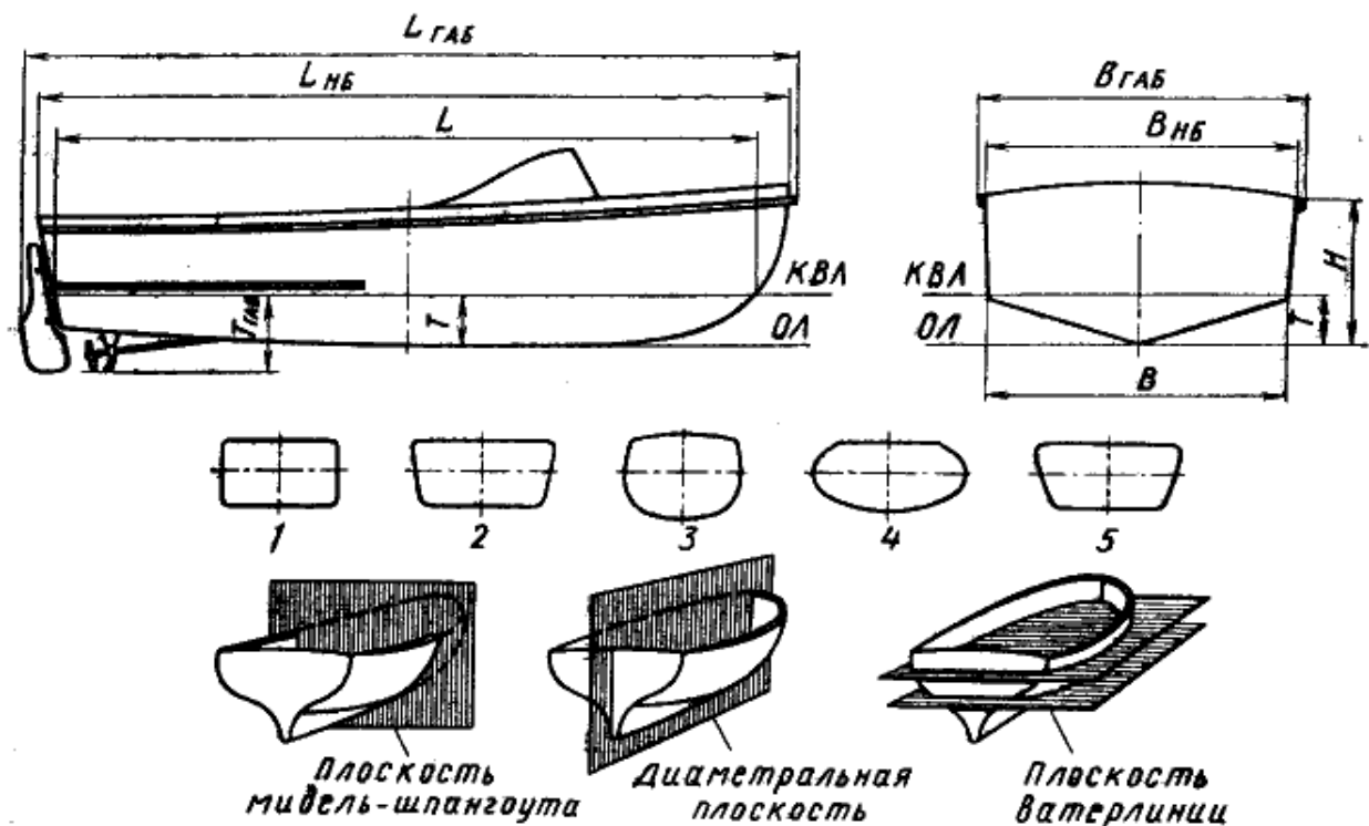
Рис. 6. Главные размеры и сечения корпуса, 1, 2, 3, 4, 5 — сечения по плоскости мидель-шпангоута судов различных типов
