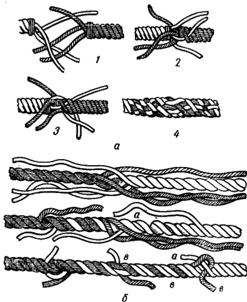
Рис. 154. Спlesenь: a — короткий спlesenь (1—4 — последовательные приемы сращивания двух тросов); б — длинный спlesenь
