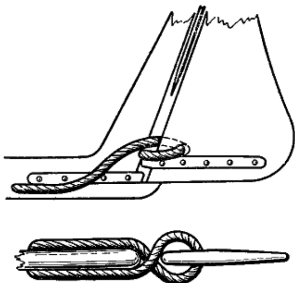
Рис. 135. Замена петель руля
