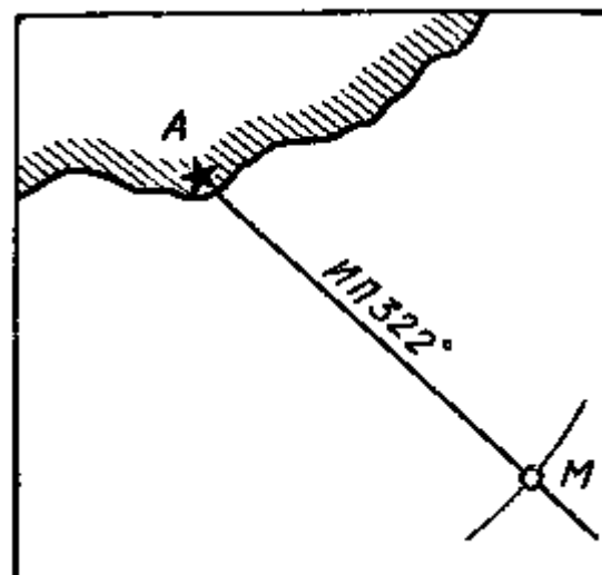
Рис. 47. Определение места судна по пеленгу предмета и расстоянию до него
