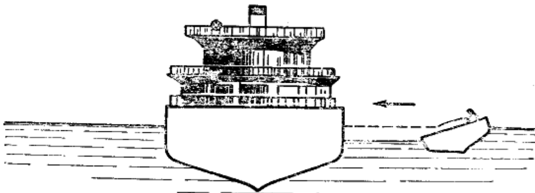
Рис. 108. Подсасывание малого судна к большому
