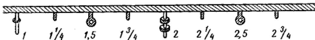
Рис. 70. Схема разбивки лаглиня
