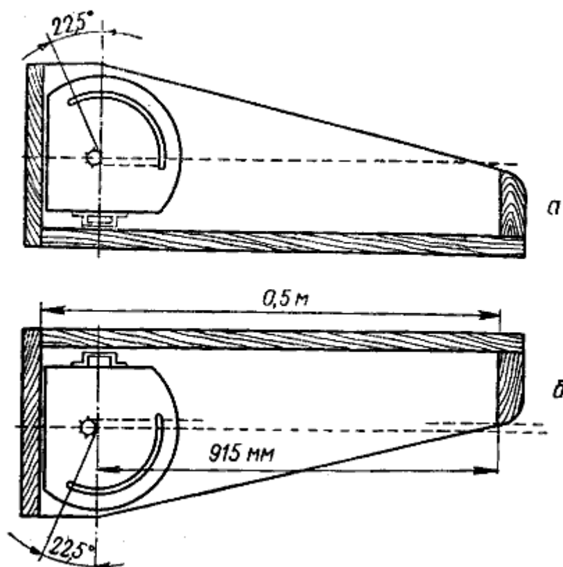
Рис. 168. Устройство отличительных бортовых сигналов: а — щит и фонарь левого борта окрашенный в красный цвет; б — щит и фонарь правого борта, окрашенный в зеленый цвет
