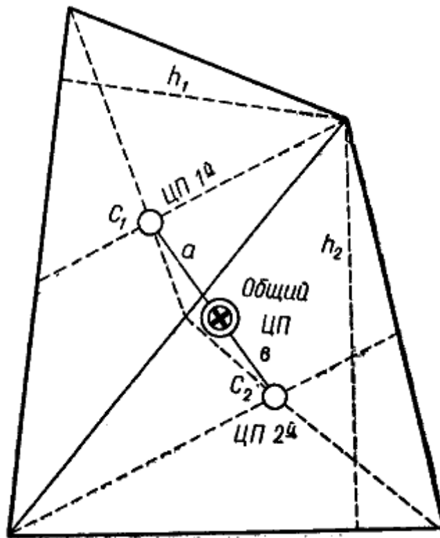
Рис. 146. Определение площади паруса
