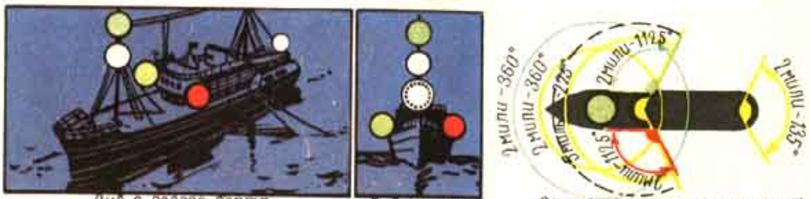
14. Судно длиной не менее 12,19 м, занятое ловом рыбы, кроме судов, занятых тралением, на ходу (правило 9,д,ф)
