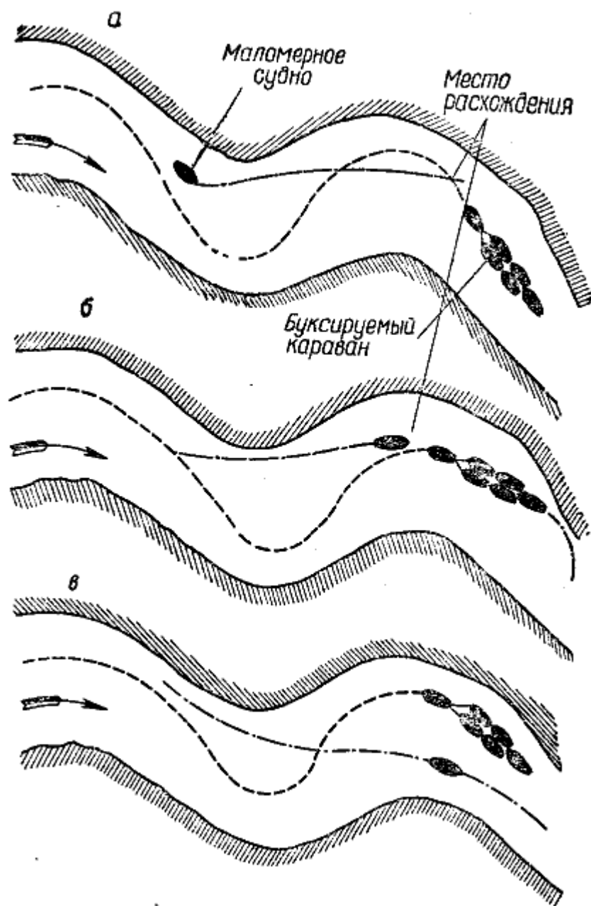
Рис. 112. Расхождение состава и катера при встрече
