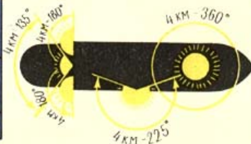
Схема расположения стояночных огней
