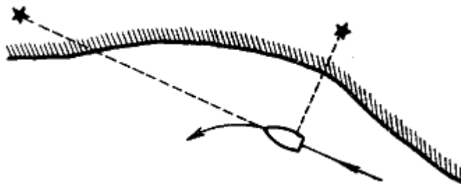
Рис. 56. Определение места судна способом прямого угла
