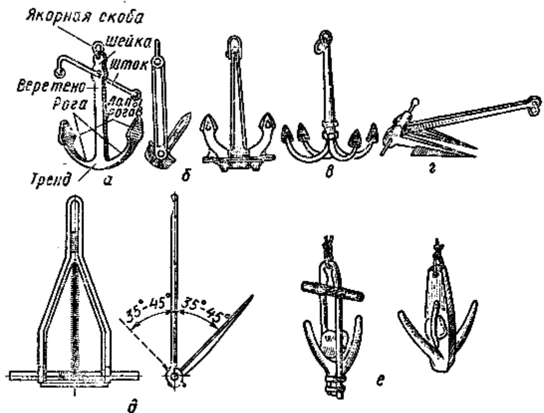
Рис. 113. Якоря а — адмиралтейский; б — Холла; в — четырехлапый; г — Матросова, д — четырехлапый сварной Курбатова; е — самодельные из дерева
