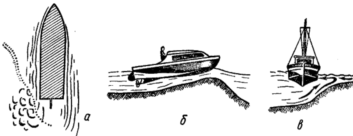
Рис. 29. Проверка правильности курса: a — по придонной волне; б — по подниманию носовой части катера; в — по рысканию судна от мели
