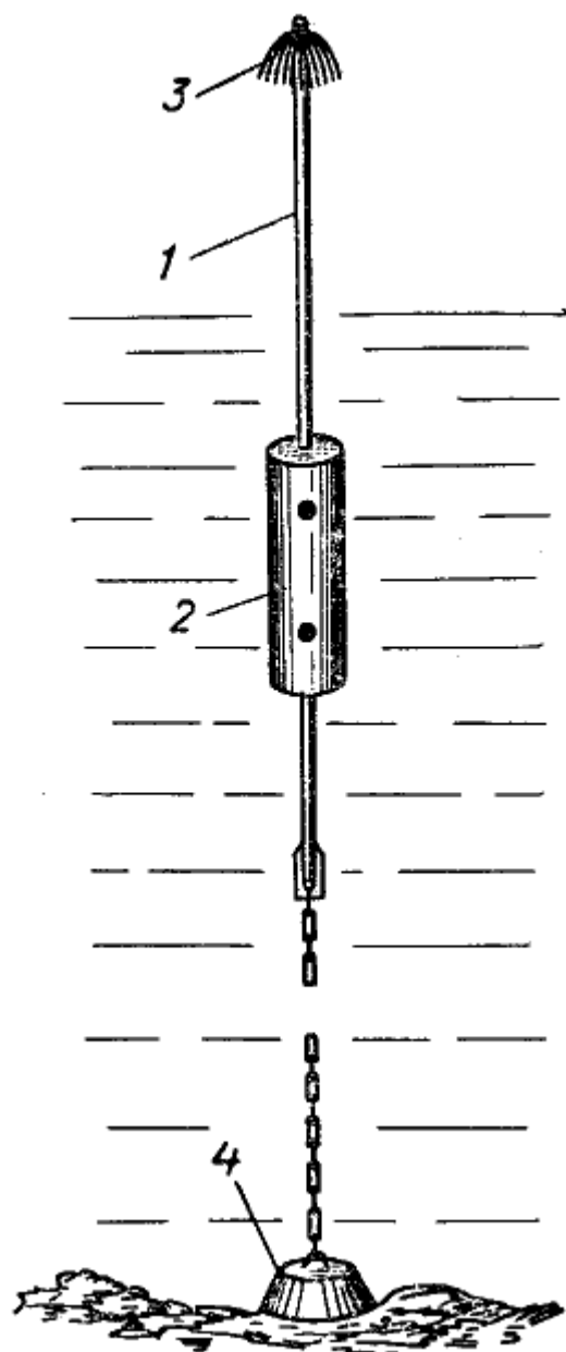
Рис. 36 Веха: 1 — деревянный шест; 2 — боек; 3 — топовая фигура; 4 — якорь
