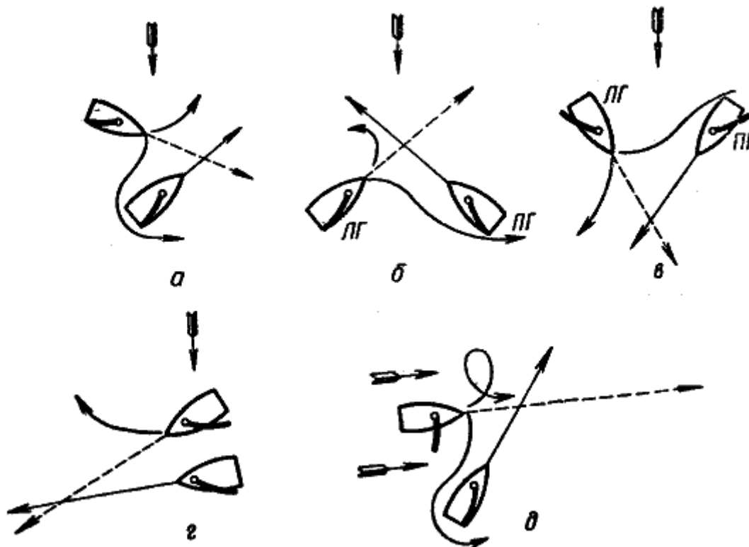
Рис. 142. Правила расхождения парусных судов
