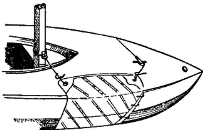
Рис. 133. Мягкий пластырь, закрепленный на пробое корпуса
