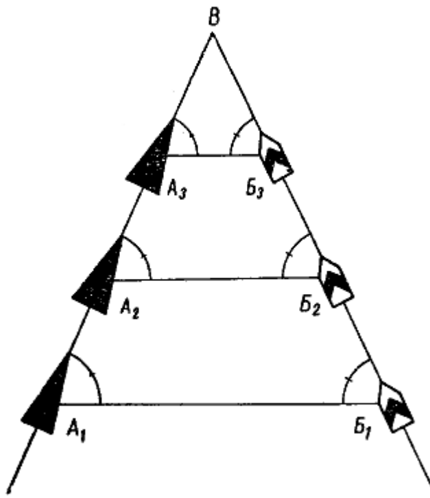
Рис. 172. Пеленг на приближающееся судно не меняется
