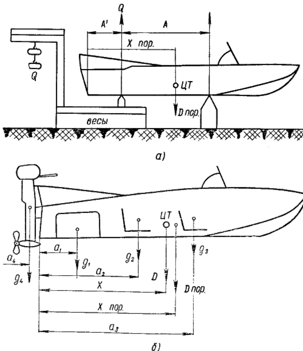
Рис. 87 а, б. Определение ЦТ путем взвешивания
