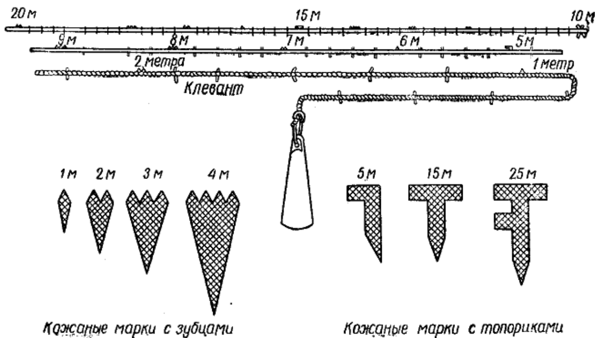
Рис. 72. Устройство и схема разбивки ручного лота
