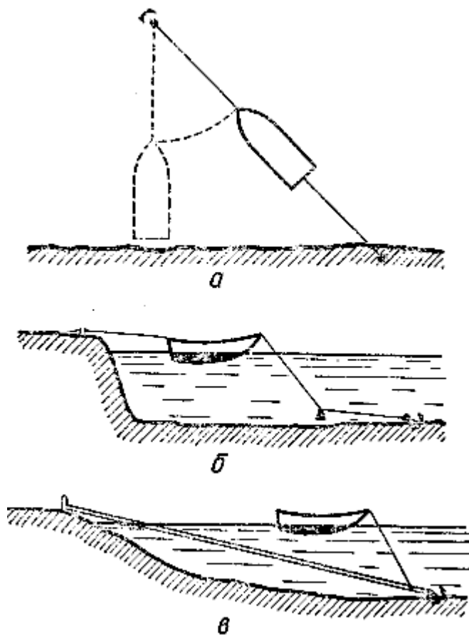
Рис. 122. Стоянка судов на якорь вблизи берега
