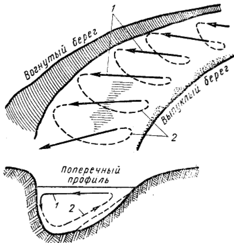
Рис. 10. Внутреннее течение на изгибе русла: 1 — направление течения на поверхности — прижимное течение; 2 — направление течения на дне — донное течение
