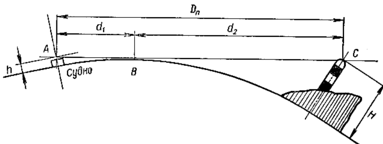
Рис 39. Дальность видимости предмета
