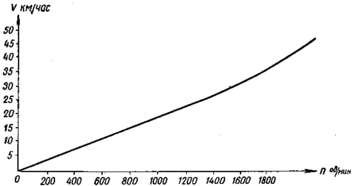
Рис. 60. График зависимости скорости судна от числа оборотов двигателя
