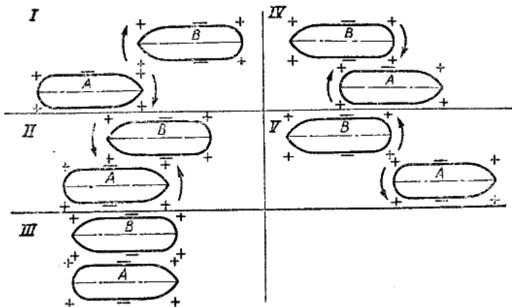
Рис. 106. Взаимодействие между судами, расходящимися на близком расстоянии друг от друга. Стрелками показано направление оконечностей судна
