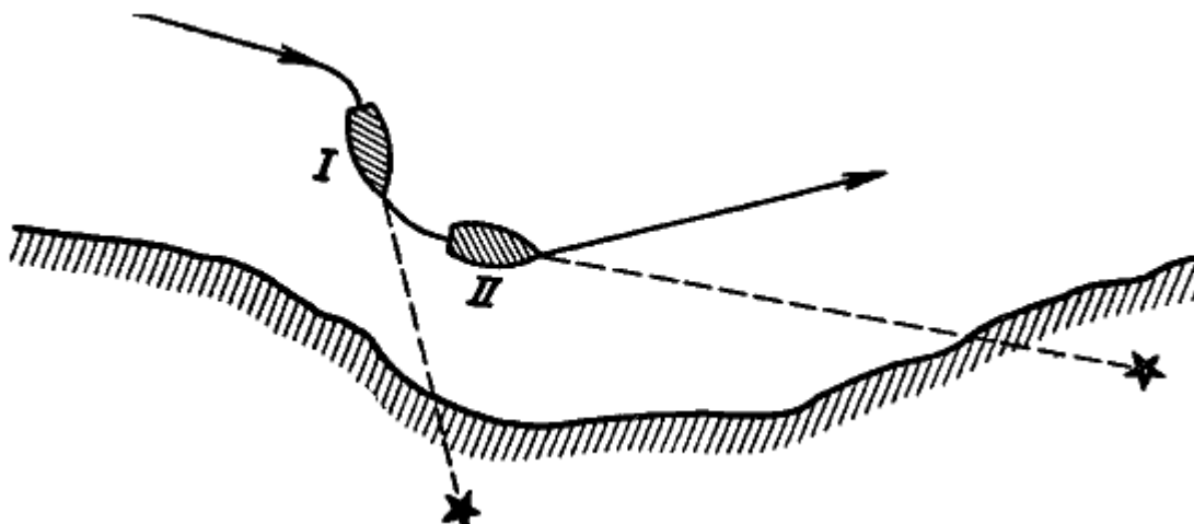
Рис. 55. Определение места судна способом двух последовательных курсов
