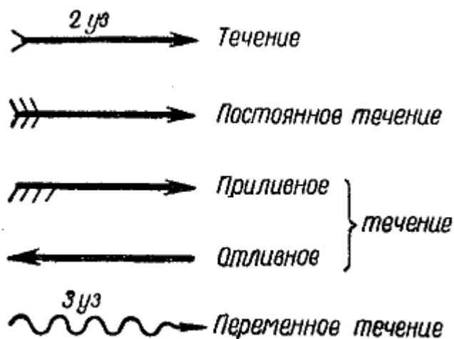
Рис. 81. Обозначение течений на картах и в атласах
