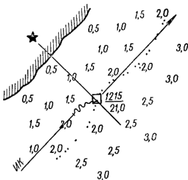
Рис. 52 Опознание места судна по пеленгу и глубине
