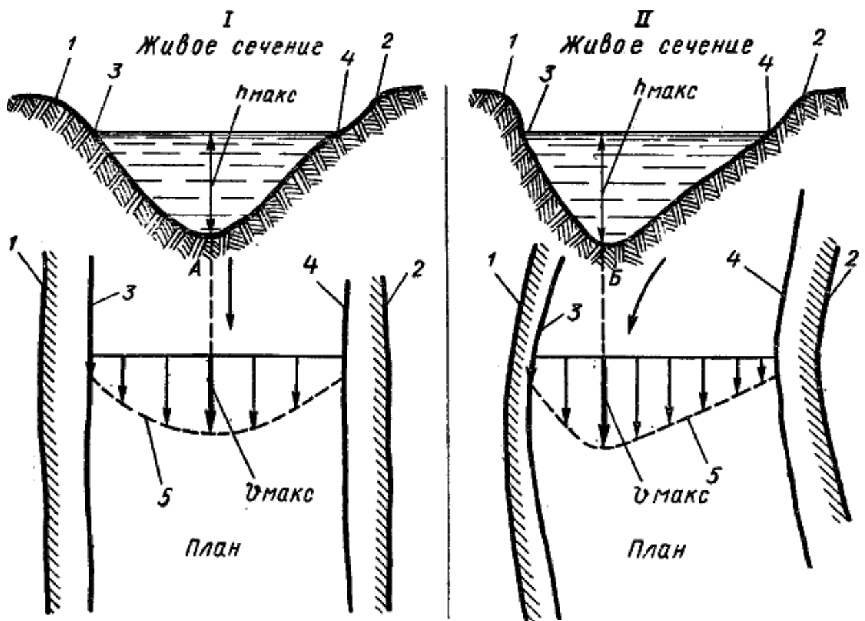
Рис. 9. Распределение поверхностных скоростей течения в плане: / — симметричное русло; II — несимметричное русло. 1 — бровка правого берега; 2 — бровка левого берега; 3 — правый урез воды; 4 — левый урез воды; 5 — распределение скоростей течения в плане
