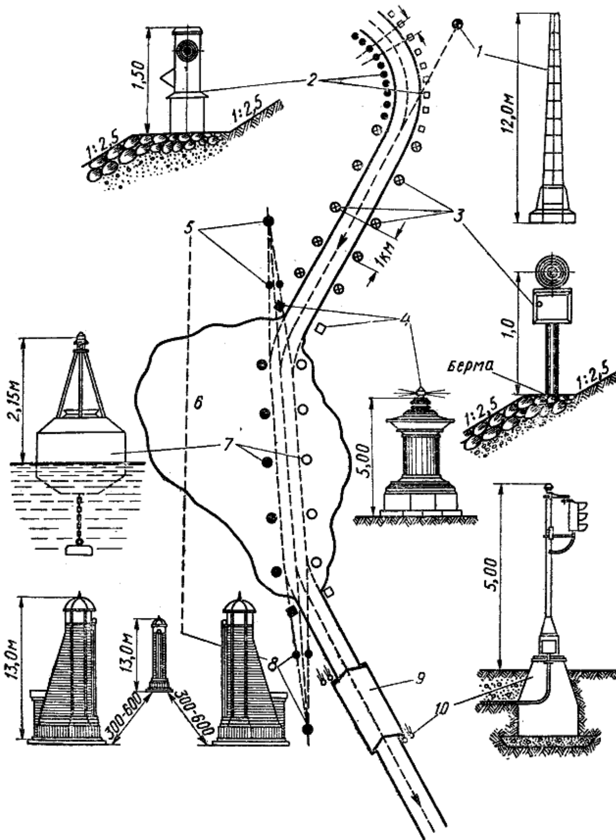
Рис. 25. Схема обстановки водохранилища и канала: 1 — прицельный знак перспективного створа; 2 — путевые огни; 3 — береговые знаки; 4 — опознавательные знаки; 5, 8 — знаки щелевого створа; 6 — водохранилище; 7 — плавучие буи; 9 — шлюз; 10 — светофор
