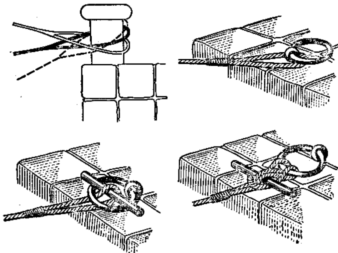
Рис. 123. Крепление швартовых тросов на берегу
