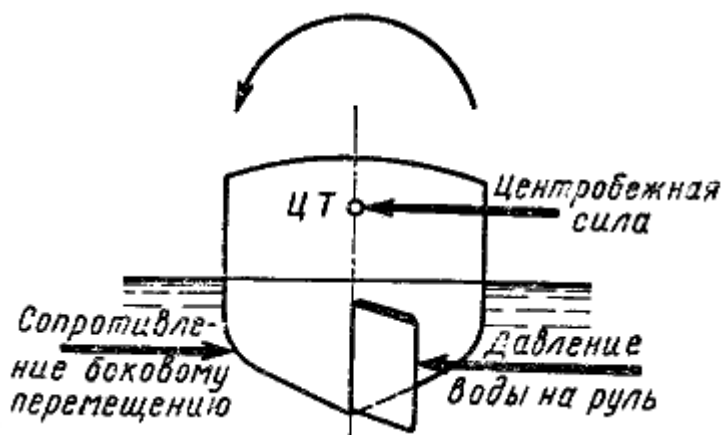
Рис. 98 Силы, выбывающие крен на циркуляцию
