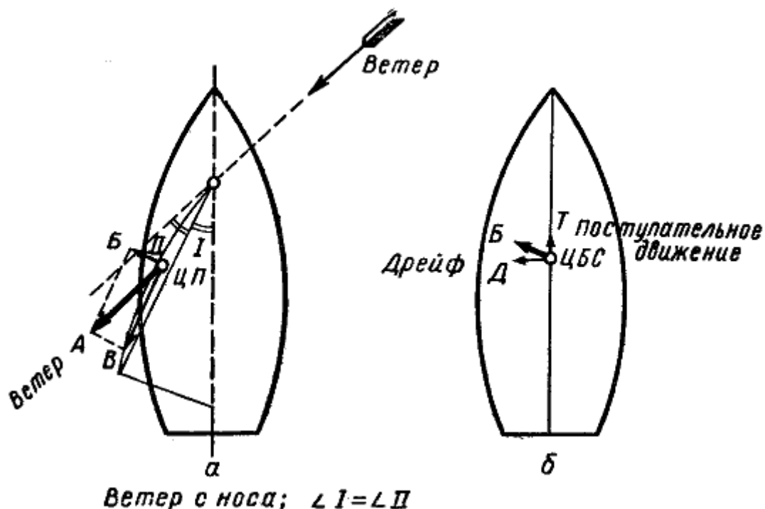
Рис. 137. Силы, действующие на парус и судно при ветре с носовых углов
