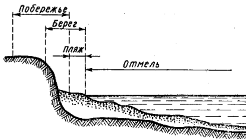
Рис. 31. Элементы береговой зоны
