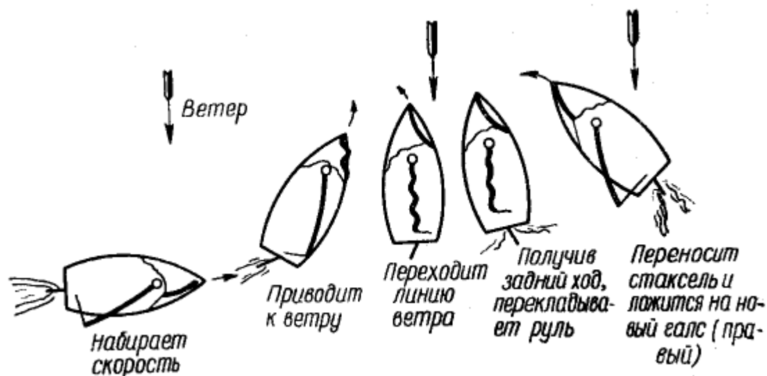
Рис 140. Поворот оверштаг
