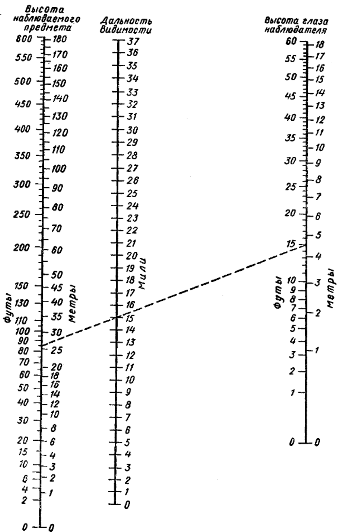
Рис. 40. Номограмма Струйского
