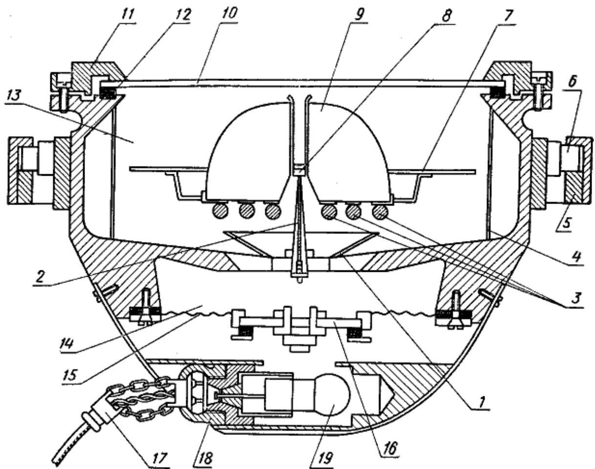
Рис. 63. 127-миллиметровый компасный котелок с донным освещением системы ГУ: 1 — отражатель света; 2 — шпилька; 3 — магнитные стрелки; 4 — курсовая черта; 5 — карданное кольцо; 6 — цапфа; 7 — картушка; 8 — топка; 9 — поплавок; 10 — стекло; 11 — азимутальный круг; 12 — резиновая прокладка; 13 — верхняя камера; 14 — нижняя камера; 15 — диафрагма; 16 — световое окно; 17 — кольцо для вытаскивания патрона; 18 — патрон; 19 — электрическая лампочка
