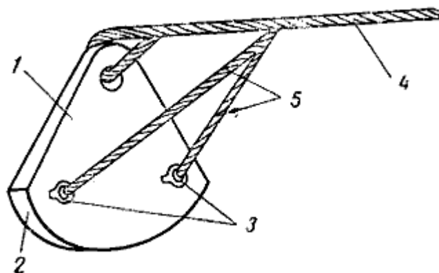
Рис. 71. Ручной лот 1 — сектор; 2 — свинцовая пластина; 3—клеванты; 4 — лаггиль; 5 — путики
