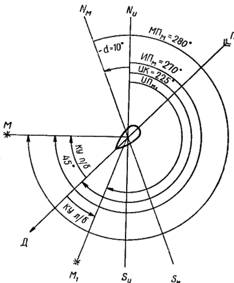
Рис. 42. Определение истинного пеленга через курсовой угол или склонение
