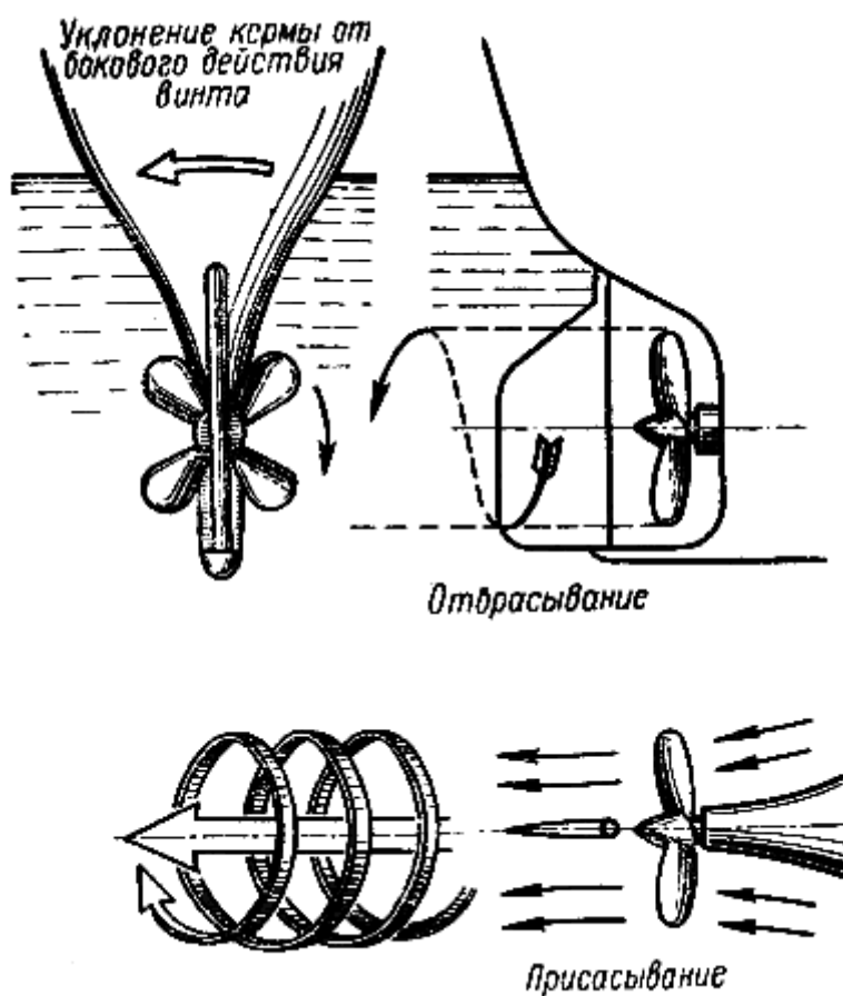
Рис. 103. Образование потоков винтов
