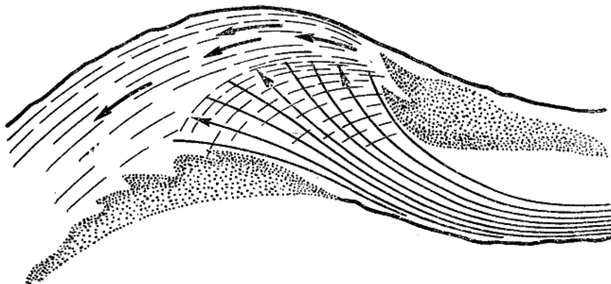
Рис. 18. Течение на перекале с выпуклым подвальем
