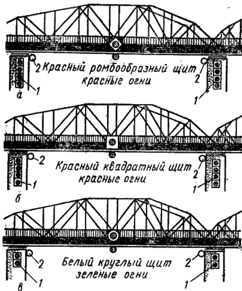
Рис. 24. Сигнализация на железнодорожных и шоссейных мостах: а — обстановка судоходного пролета сверху; б — обстановка судоходного пролета снизу; в — обстановка пролета для сплава; 1 — зеленые огни; 2 — белые огни для освещения опор моста
